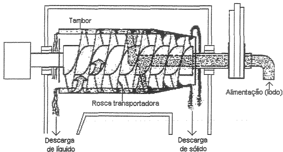
FIGURA 7 – Centrífuga Contracorrente (desenho esquemático)
