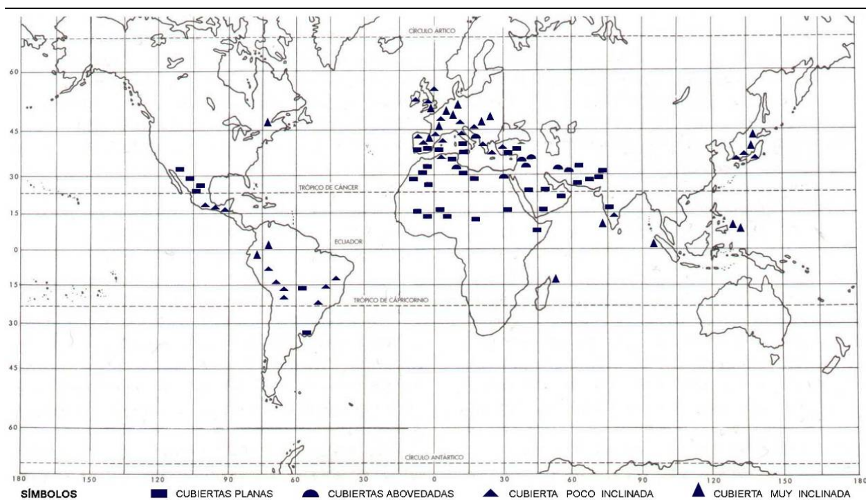
Fig. 5 Classificação das coberturas vernáculas segundo a zona climática
