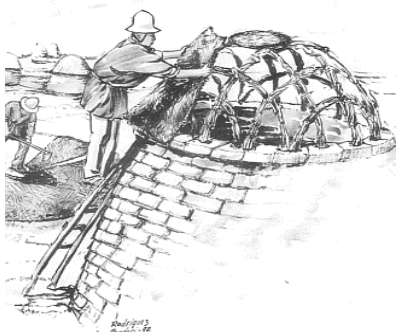
Fig. 52 Componentes construtivos da moradia Chipaya
