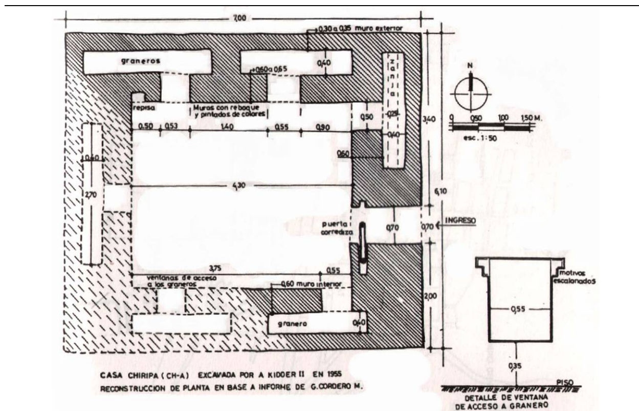
Fig. 30 Moradias de parede dupla dos Chiripas
