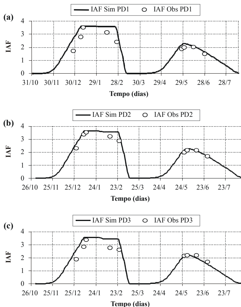
Figura 4.33. Índice de área foliar (IAF) observado com o uso do LAI 2000 e simulado pelo modelo STICS para a sequência das culturas do milho, variedade Cargil 901 e do milheto, variedade BRS 1501, nas parcelas cultivadas no sistema de plantio direto: PD1 (a), PD2 (b) e PD3 (c).
