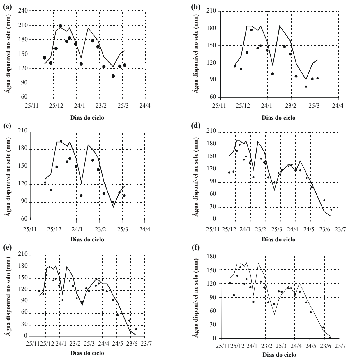
Figura 4.34. Comparação dos valores observados (• • • •) e simulados (—) da água disponível no solo (mm) até 180 cm de profundidade, durante o ciclo da cultura do milho, no sistema de manejo convencional PC1 (a), PC2 (b) e PC3 (c), e da seqüência milho-milheto no sistema de plantio direto PD1 (d), PD2 (e) e PD3 (f).
