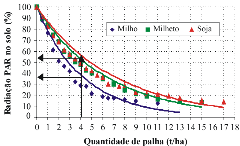
Figura 4.7. Ajuste da porcentagem da radiação PAR em função da quantidade (t/ha) de palha de milho, milheto e soja.
