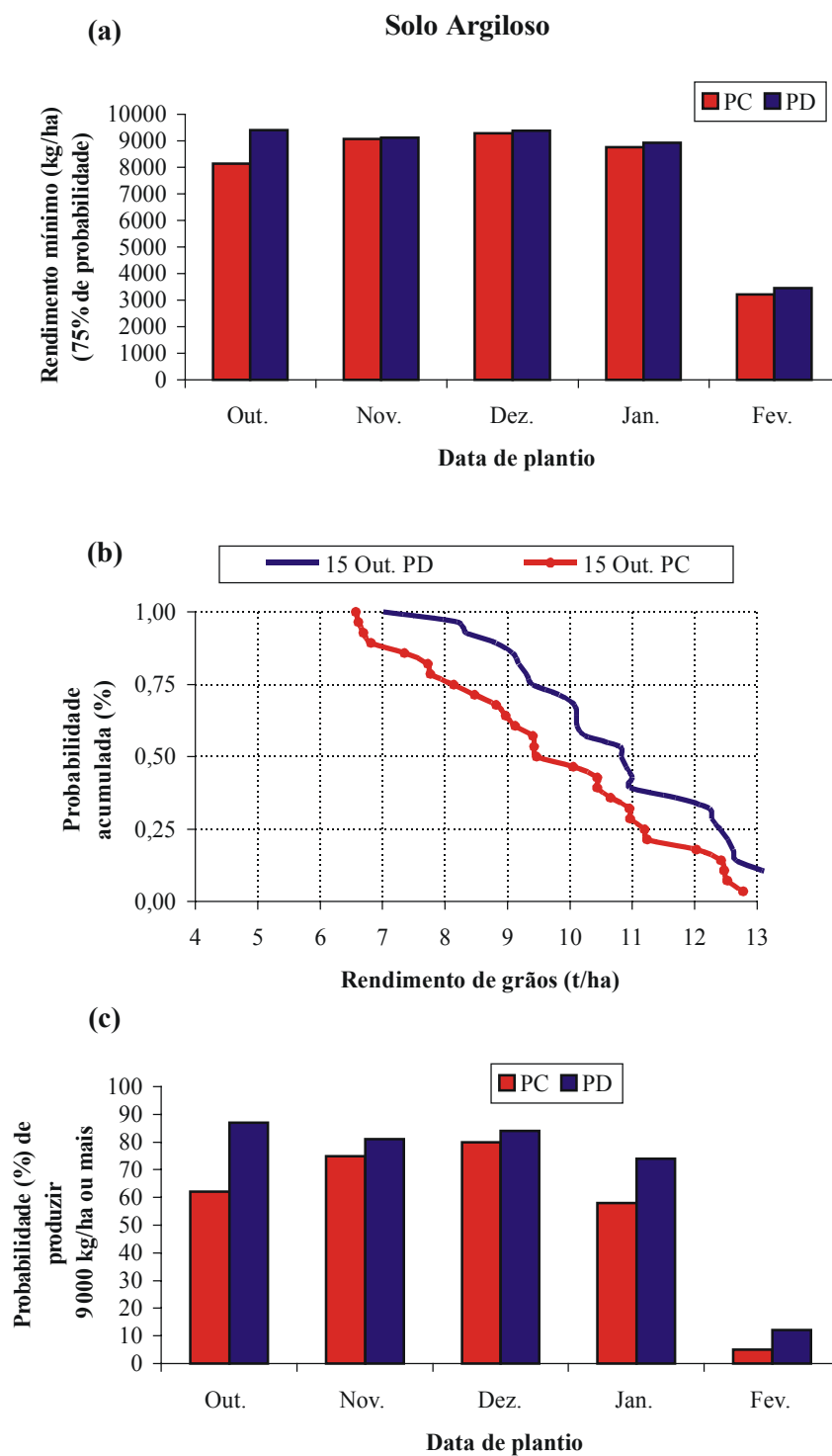
Figura 4.55. Rendimento mínimo ( \text{kg} \cdot \text{ha}^{-1} ) do milho ao nível de 75% de probabilidade (a), curvas das freqüências acumuladas (%) para o plantio em 15 de outubro (b) e probabilidade (%) de o rendimento do milho ser igual ou superior a 9000 \text{ kg} \cdot \text{ha}^{-1} (c), nos sistemas convencional e plantio direto, em solo argiloso, na localidade de Planaltina-DF.
