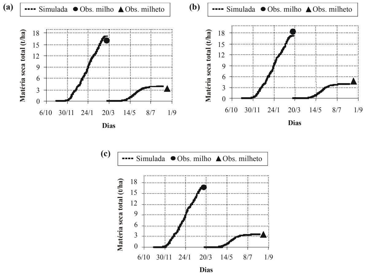
Anexo 4.20. Matéria seca total observada e simulada das culturas do milho, variedade cargil 901, e do milheto, variedade BRS 1501, nas parcelas PD1, (a), PD2 (b) e PD3 (c) do sistema de manejo plantio direto.
