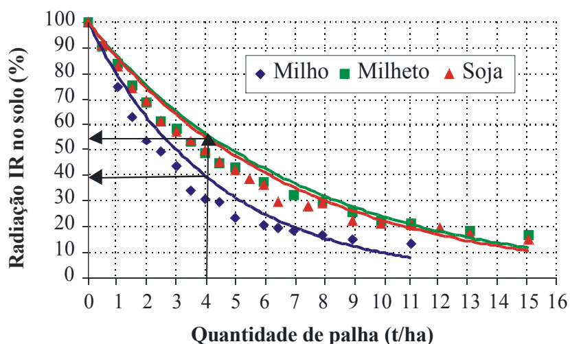
Figura 4.8. Ajuste da porcentagem da radiação IR em função da quantidade (t/ha) de palha de milho, milheto e soja.
