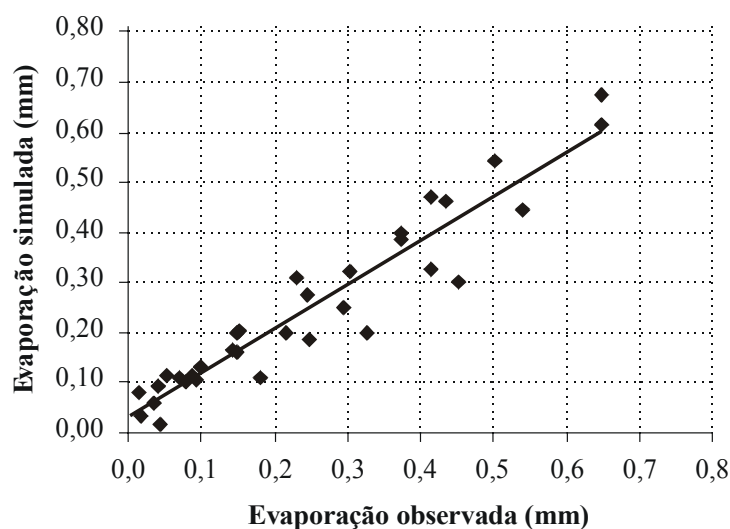
Figura 4.18. Relação entre a evaporação observada (mm) e a simulada (mm) para diversas quantidades de palhada de milho.
