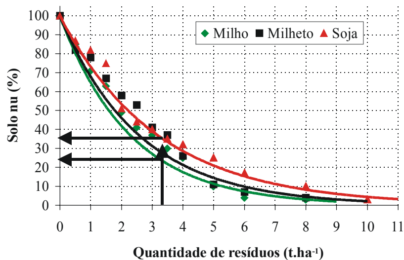
Figura 4.4. Ajuste exponencial entre taxa de cobertura (TC, %) e quantidade (t/ha) de palha de milho, milheto e soja.
