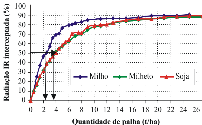
Figura 4.6. Porcentagem da radiação IR interceptada em função da quantidade (t/ha) de resíduos de milho, milheto e soja.
