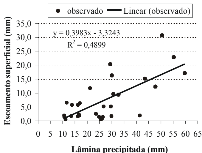
Figura 4.22. Coeficiente de determinação ( R^2 ) e modelo de ajuste linear (y) entre lâminas escoadas (mm) observadas no sistema convencional.
