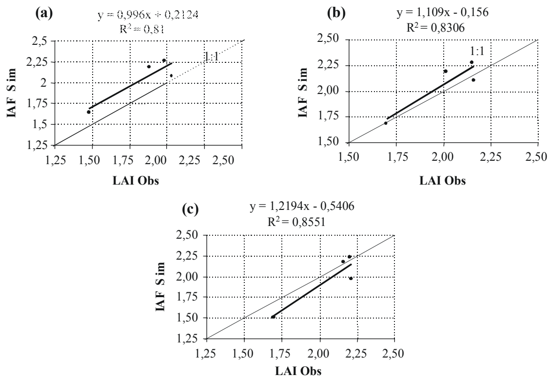
Anexo 4.16. Comparação entre índice de área foliar (IAF) observado e simulado para a cultura do milho, variedade BRS 1501, nas parcelas PD1 (a), PD2 (b) e PD3 (c) do sistema de plantio direto.
