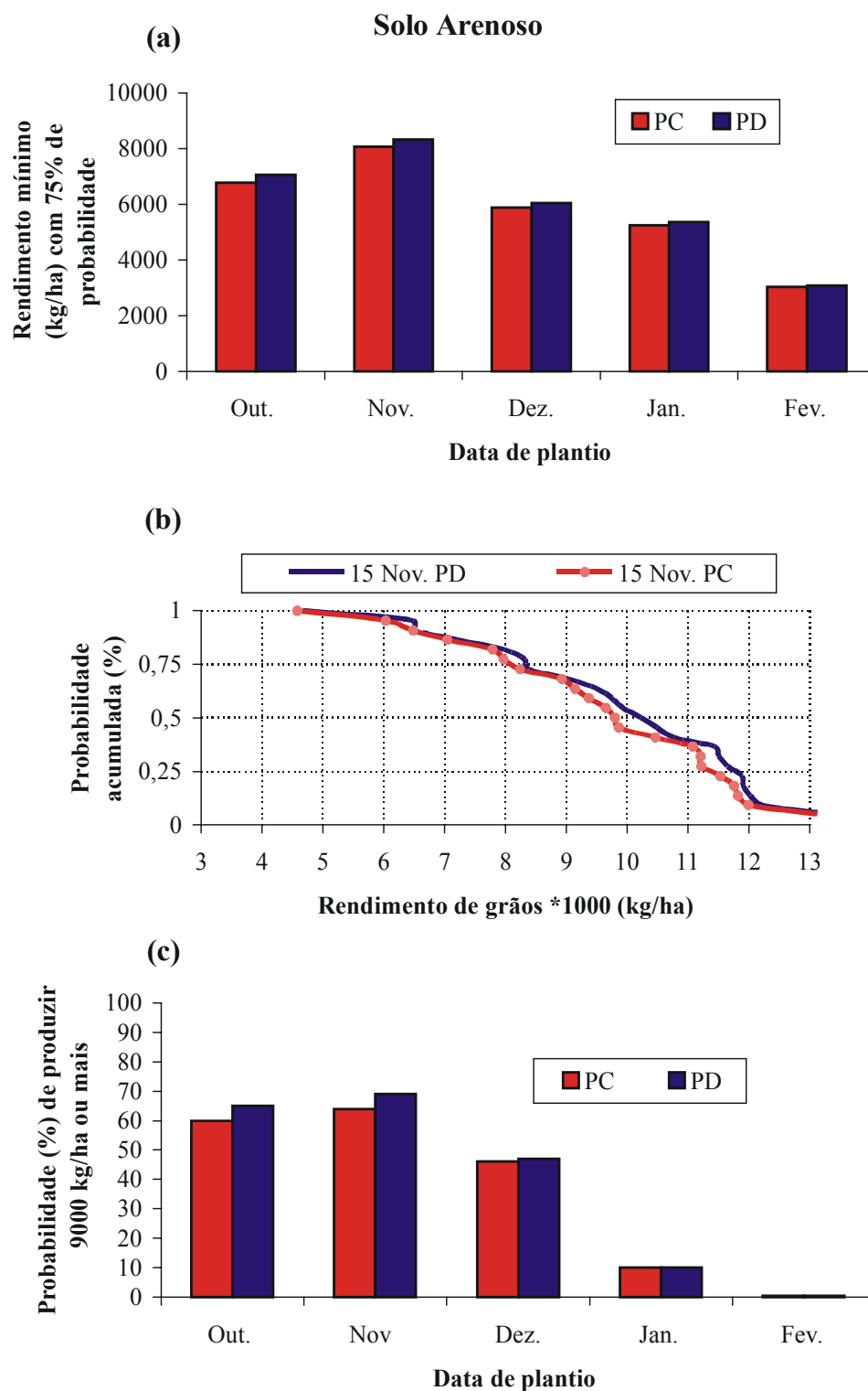
Figura 4.56. Rendimento mínimo ( \text{kg} \cdot \text{ha}^{-1} ) do milho ao nível de 75% de probabilidade (a) , curvas das freqüências acumuladas (%) para o plantio em 15 de outubro (b) e probabilidade (%) de o rendimento do milho ser igual ou superior a 9000 \text{ kg} \cdot \text{ha}^{-1} (c) , nos sistemas convencional e plantio direto, em solo textura média, na localidade de Passo Fundo-RS.
