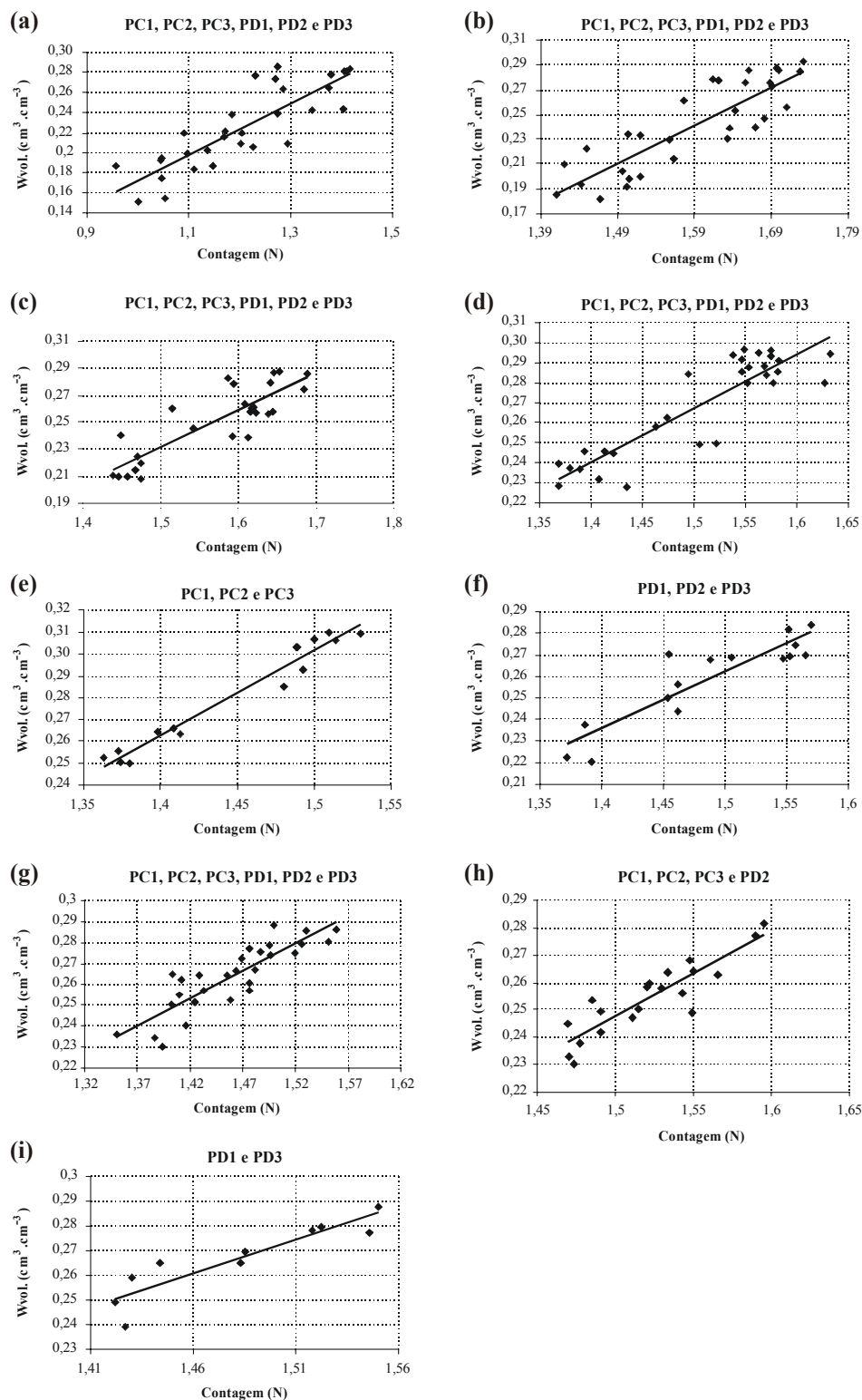
Anexo 4.17. Ajuste dos dados de umidade volumétrica do solo ( W_{vol} - \text{cm}^3 \cdot \text{cm}^{-3} ) e de contagem da sonda de nêutrons N (—), mediante análise de regressão linear simples, para as profundidades: 10 cm (a); 20 cm (b); 40 cm (c); 60 cm (d); 80 cm (e) e (f), 100 cm (g), 120 cm (h) e (i), nos sistemas de manejo convencional (PC) e plantio direto (PD).
