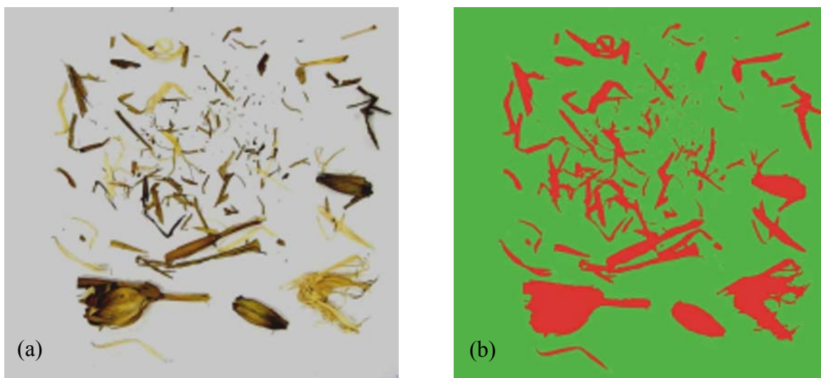
Figura 4.2. Foto de 0,5 tonelada de palha de milho (a) adquirida por máquina digital e imagem classificada pelo método da máxima verossimilhança (b) indicando uma cobertura de 16% do solo.
