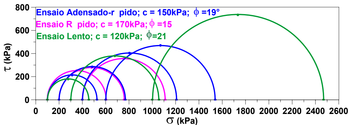
FIGURA 71 - Resultados dos ensaios triaxiais - PIT III, Prof. 8,80m – Politécnica – USP
