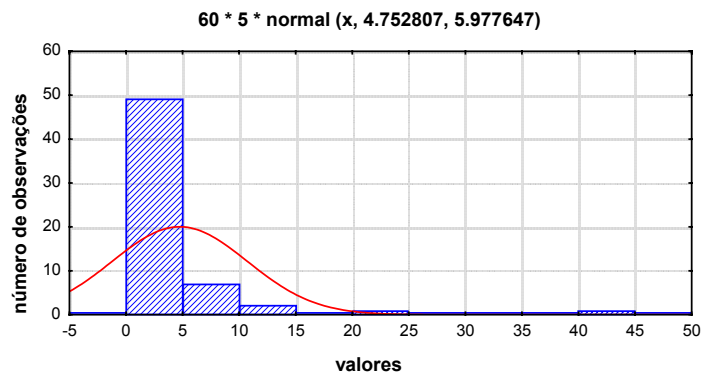
FIGURA 131 - Relação T_{Emax}/T_{ERes} para areia fina média argilosa, porosa - Unesp - Bauru
