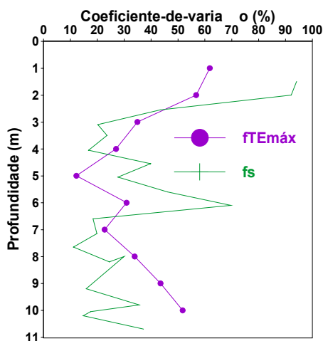
c.v. para fs e fTE máx
