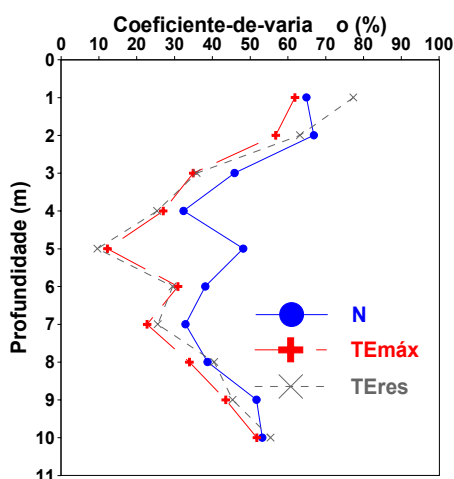
c.v. para N , TEmáx e TEres
