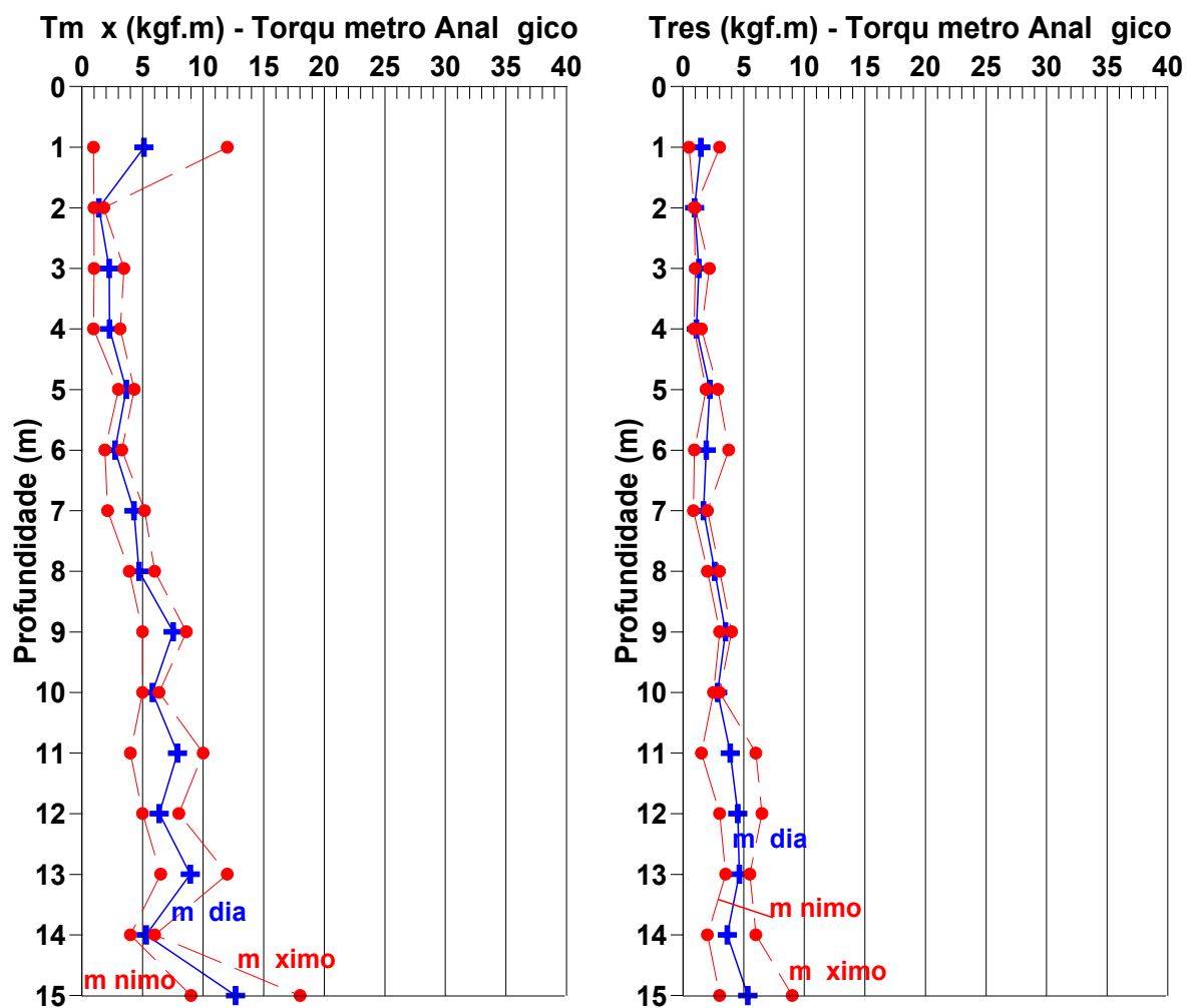
FIGURA 64 - Valores médios, máximos e mínimos de T_{m\acute{a}x} e T_{res} obtidos através do torquímetro analógico – Unesp – Ilha Solteira
