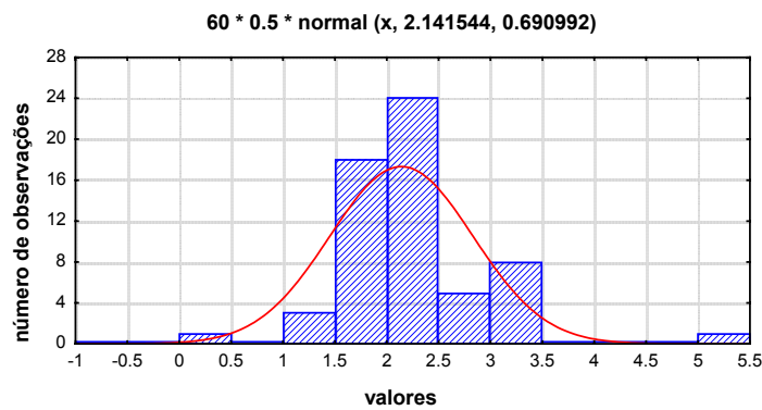
FIGURA 132 - Relação T_{máx}/T_{res} para areia fina média argilosa, porosa Unesp - Bauru
