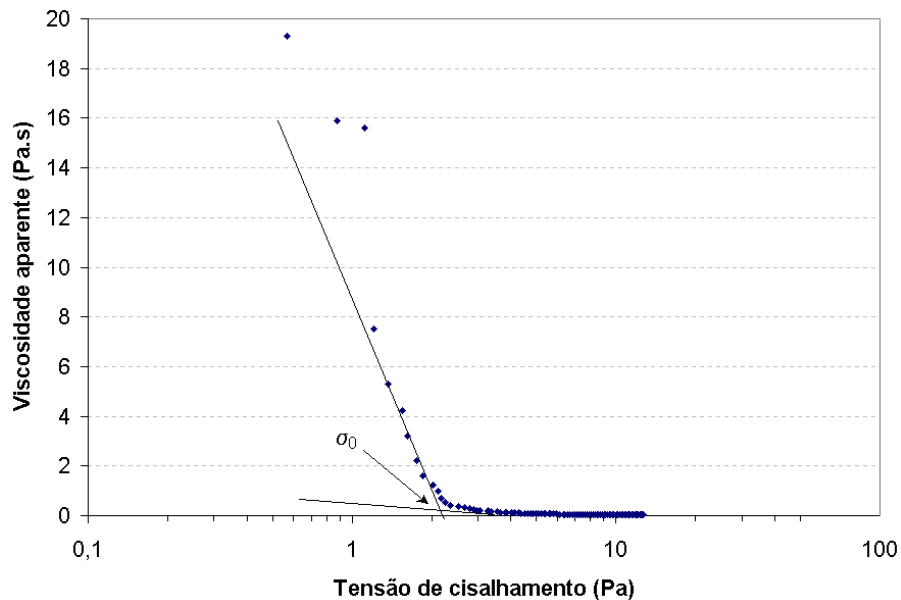
Figura 5.25 – Determinação da tensão residual através da curva de viscosidade aparente versus tensão de cisalhamento, extrapolada à viscosidade infinita
