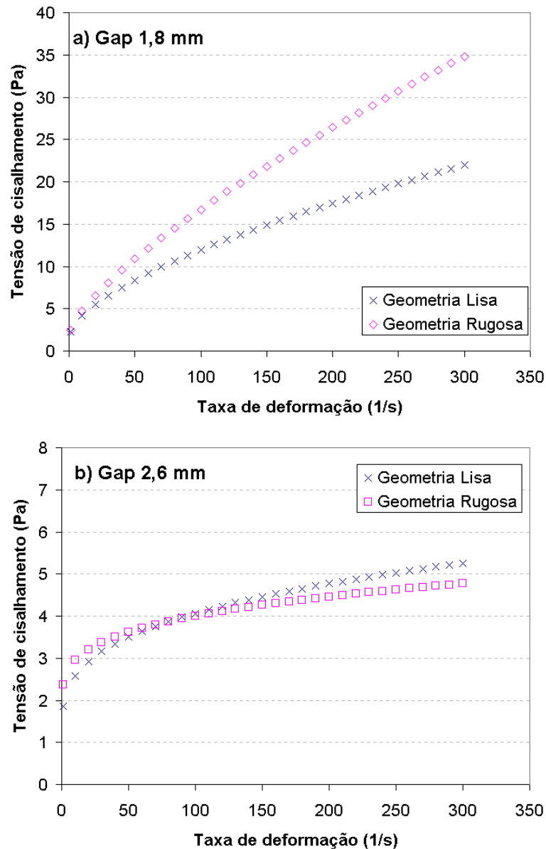
Figura 5.5 – Comparação das curvas de escoamento obtidas com geometrias de superfícies lisa e rugosa a diferentes “gaps”: a) 1,8 mm; b) 2,6 mm.
