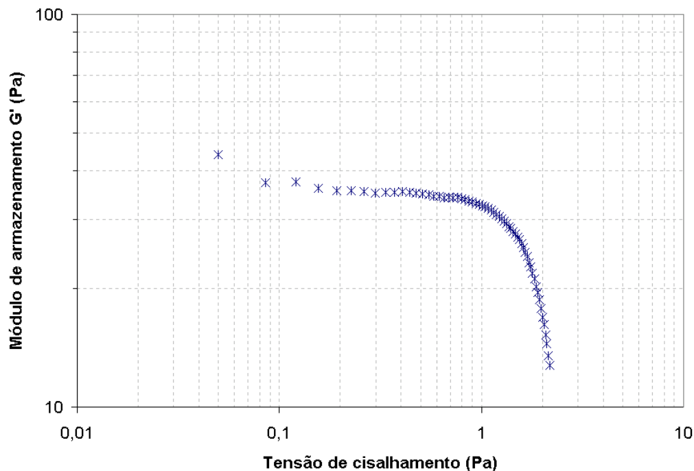
Figura 5.10 – Curva de varredura de tensão para determinação do intervalo de viscoelasticidade linear da polpa de jabuticaba.
