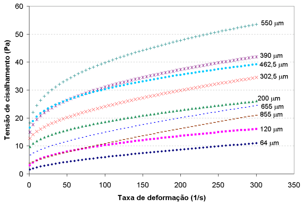
Figura 5.17 – Curvas de escoamento das amostras reconstituídas com as diferentes frações de tamanho de partículas.
