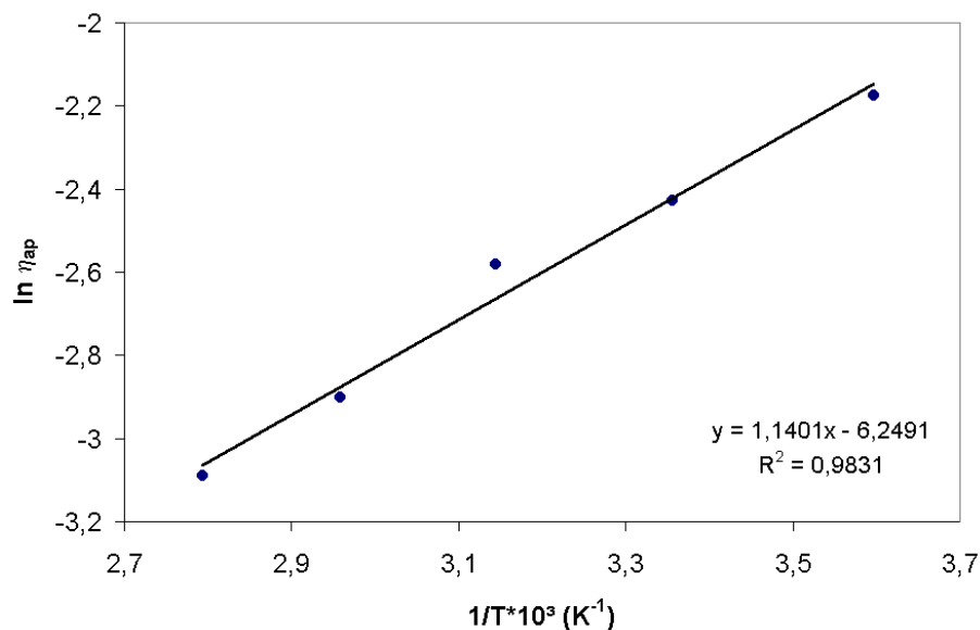
Figura 5.8 – Efeito da temperatura sobre a viscosidade aparente ( 100 \text{ s}^{-1} ) da polpa de jabuticaba.
