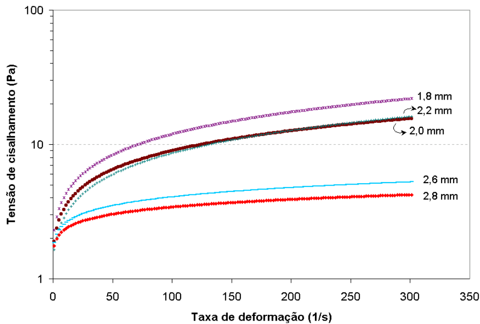
Figura 5.3 – Curvas de escoamento para diferentes gaps utilizando a geometria de superfície lisa.
