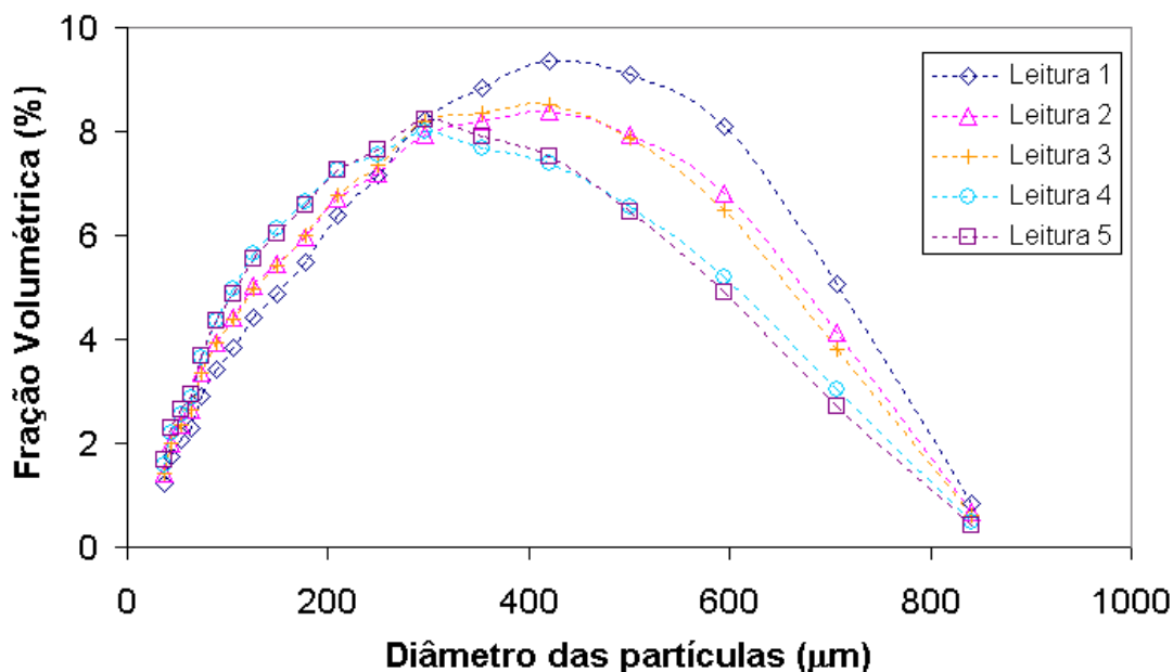
Figura 5.1 – Curvas de distribuição do tamanho de partículas dispersas com ultra-som.
