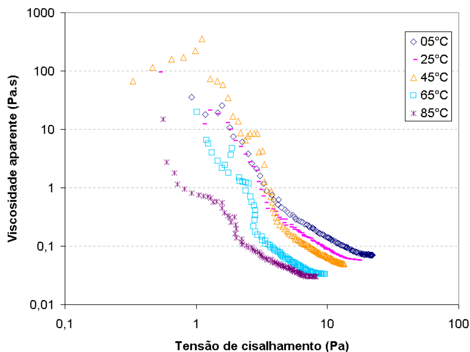
Figura 5.7 - Curva de escoamento da polpa de jabuticaba nas diferentes temperaturas.
