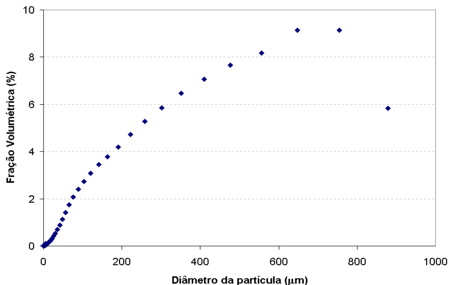
Figura 5.2 – Curva de distribuição do tamanho de partículas da polpa de jabuticaba.
