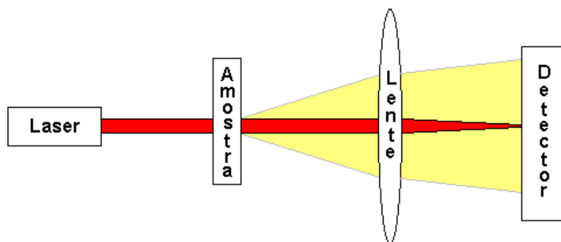
Figura 3.6 – Esquema óptico para determinação do tamanho de partículas por difração a laser.
