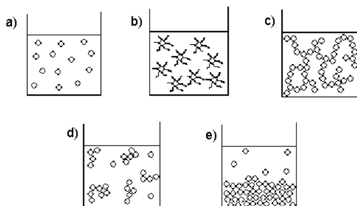
Figura 3.2 – Estrutura das partículas em uma suspensão. (a) diluídas sem interação entre as partículas; (b) estabilizadas estericamente; (c) floculadas; (d) parcialmente estáveis com alguma estrutura formada; (e) sedimentando.
