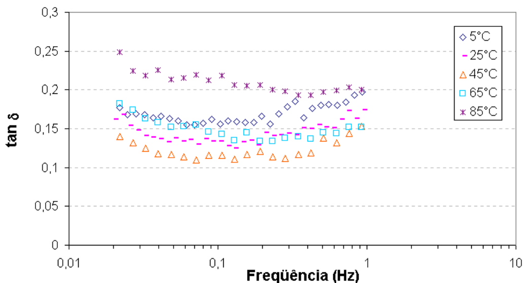
Figura 5.14 – Tangente do ângulo de fase ( \tan \delta ) em função da frequência a diferentes temperaturas.
