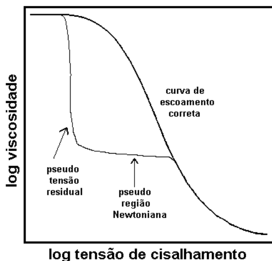
Figura 3.10 – Efeito do escorregamento em uma curva de viscosidade versus tensão de cisalhamento de um líquido estruturado mostrando uma pseudo tensão residual.
