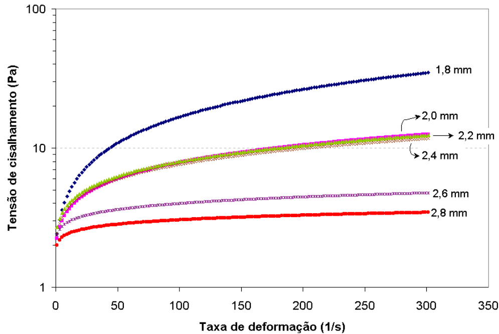
Figura 5.4 – Curvas de escoamento para diferentes gaps utilizando a geometria de superfície rugosa.
