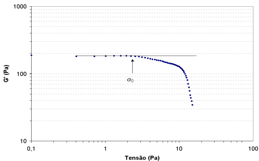
Figura 5.26 – Determinação da tensão residual através da queda do platô do módulo de armazenamento ( G' ) em função da tensão.
