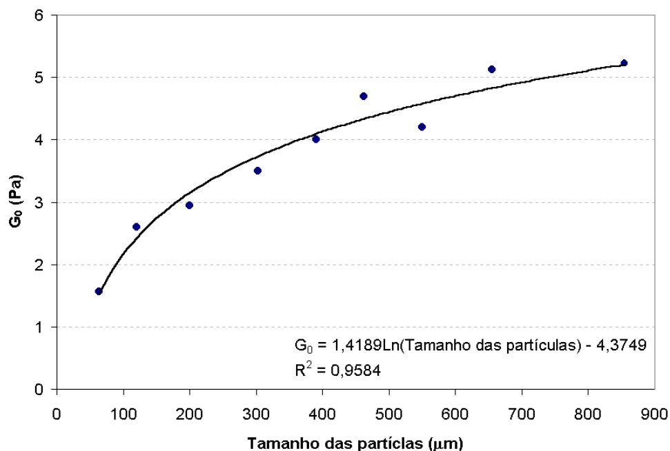
Figura 5.22 – Comportamento de G_0 em função do tamanho das partículas das amostras.
