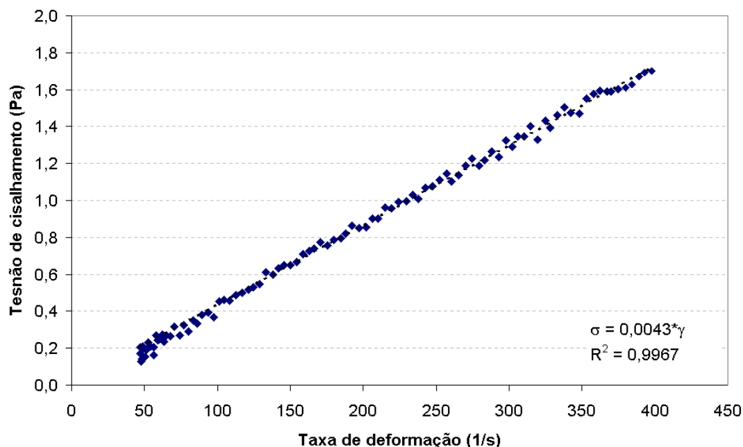
Figura 5.15 – Curva de escoamento do soro da polpa da jabuticaba.
