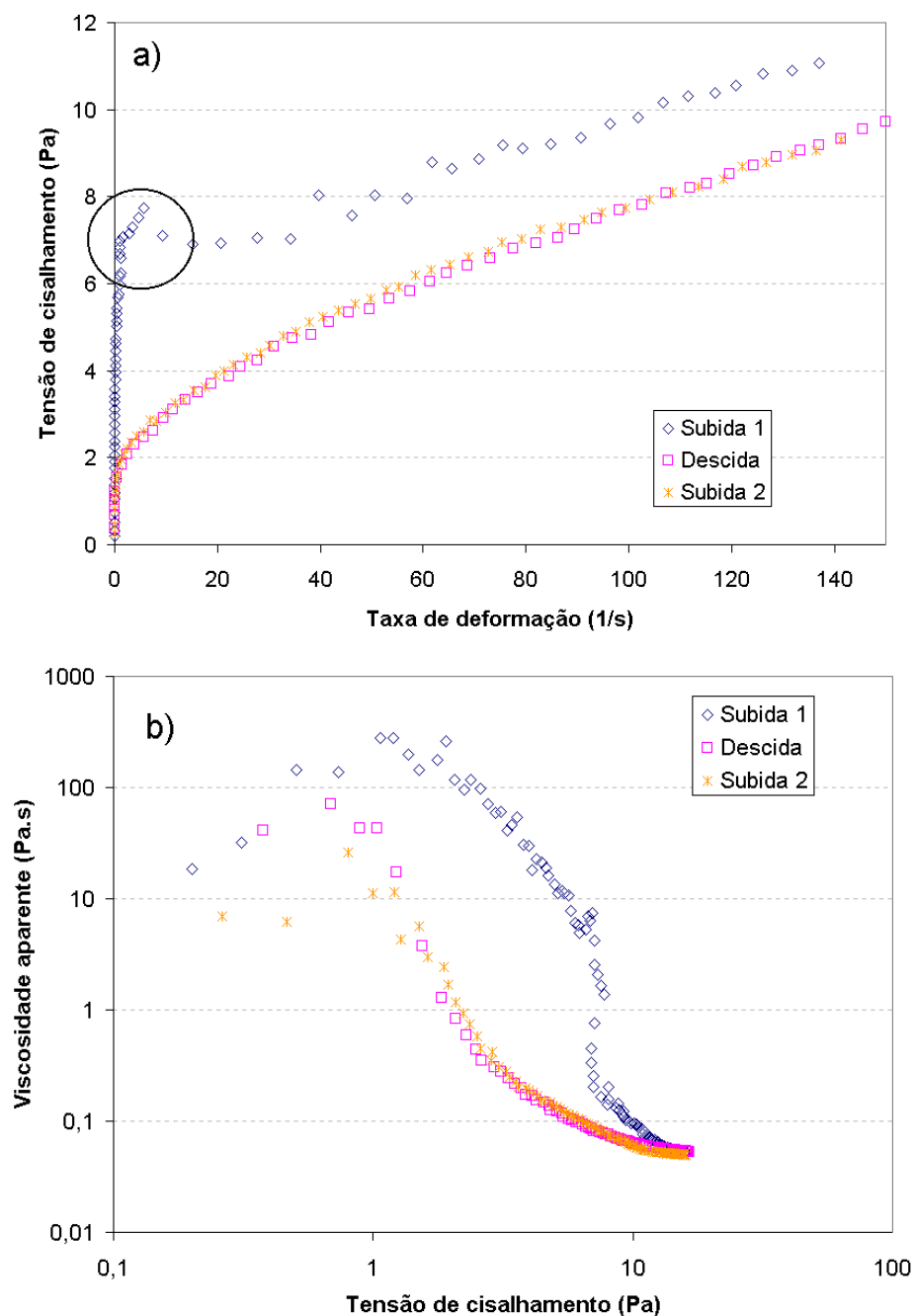
Figura 5.6 – Curva de escoamento da polpa de jabuticaba a 25 °C. a) Tensão de cisalhamento em função da taxa de deformação e b) Viscosidade aparente em função da tensão de cisalhamento.
