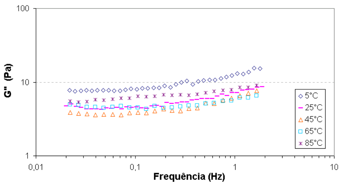
Figura 5.13 – Módulo de dissipação ( G'' ) da polpa de jabuticaba em função da frequência a diferentes temperaturas.
