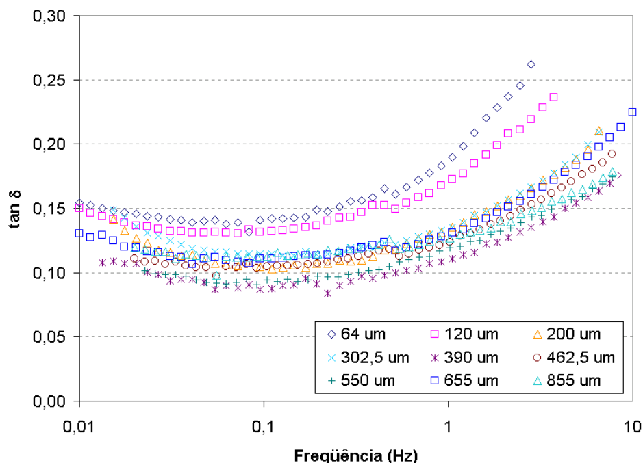
Figura 5.23 – Comportamento do ângulo de fase ( \tan \delta ) das polpas de jabuticaba reconstituídas em função da frequência das amostras com diferentes tamanhos de partículas.
