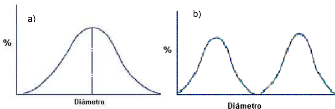
Figura 3.3 – Curvas de distribuição do tamanho de partículas de suspensões (a) monomodal; (b) bimodal.
