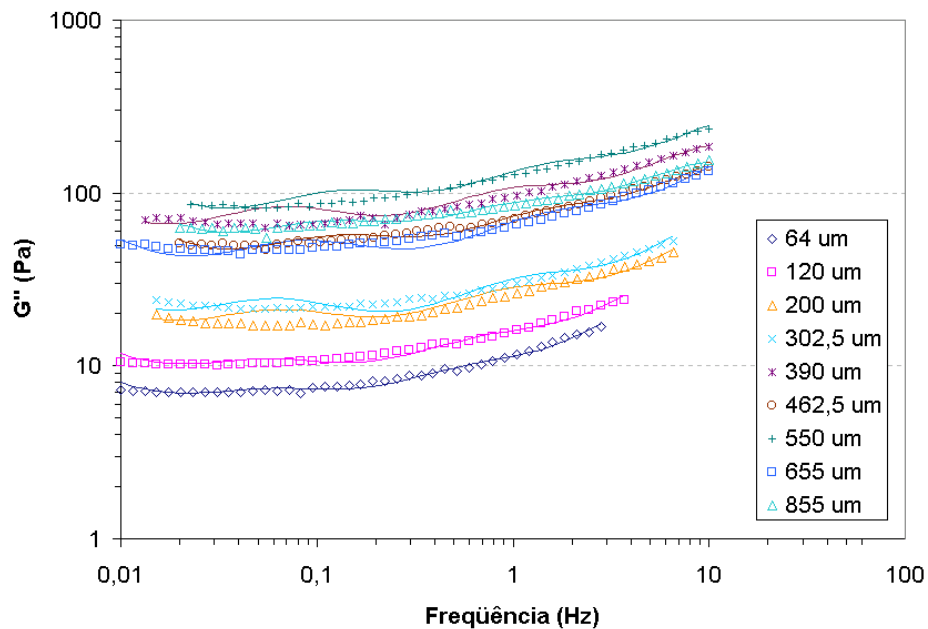
Figura 5.21 – Comportamento do módulo de dissipação ( G'' ) das polpas de jabuticaba reconstituídas em função da frequência. Linhas contínuas: dados preditos pelo modelo de Maxwell.
