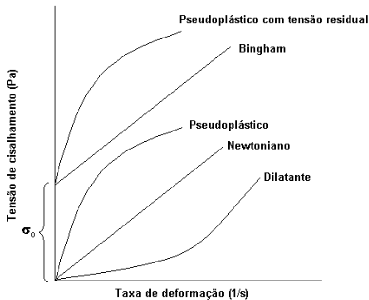
Figura 3.8 – Curvas de escoamento típicas de fluidos.
