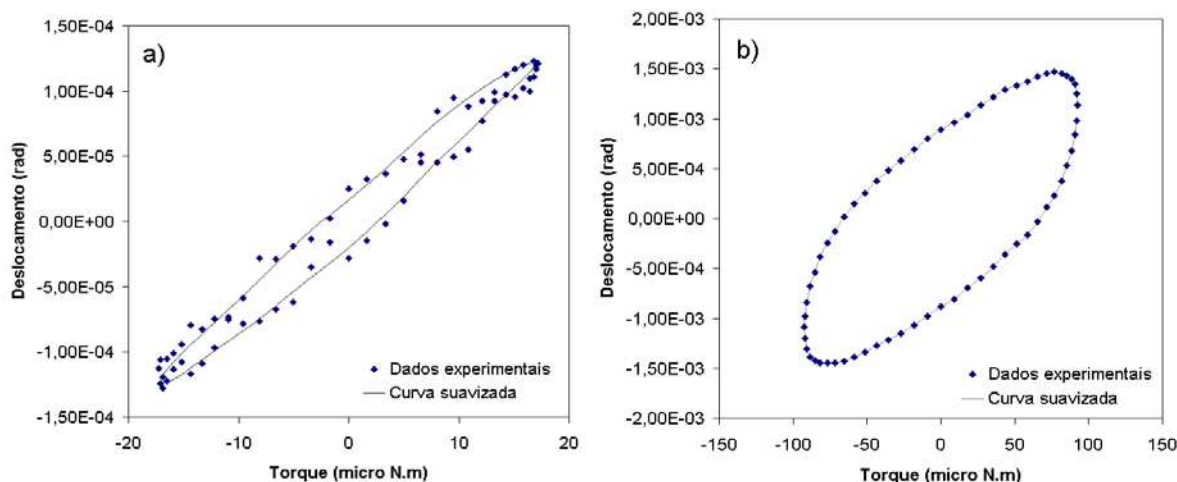
Figura 5.11- Figuras de Lissajous: (a) dentro do intervalo linear, (b) fora do intervalo linear.
