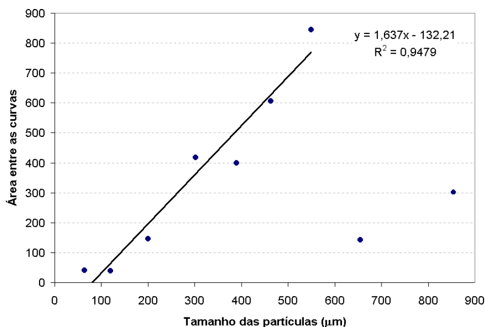
Figura 5.16 – Avaliação qualitativa da tixotropia das amostras nas diferentes condições de distribuição do tamanho de partículas.
