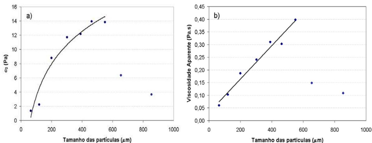
Figura 5.18 – (a) Tensão residual e (b) viscosidade aparente a 100\text{s}^{-1} em função dos diferentes tamanhos de partículas.
