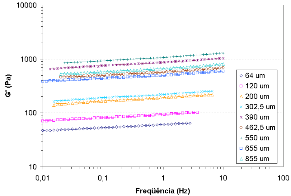
Figura 5.20 – Comportamento do módulo de armazenamento ( G' ) das polpas de jabuticaba reconstituídas em função da frequência. Linhas contínuas: dados preditos pelo modelo de Maxwell.
