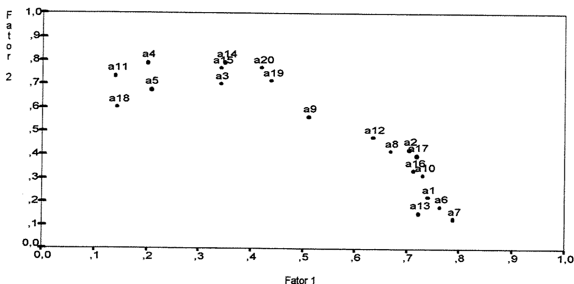
Figura 1: Gráfico de dispersão das proposições da escala de atitudes em relação à Estatística segundo as cargas fatoriais.
