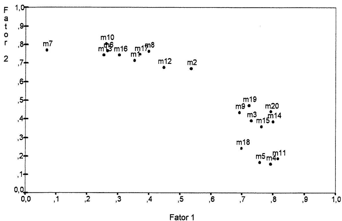
Figura 2: Gráfico de dispersão das proposições da escala de atitudes em relação à matemática, segundo as cargas fatoriais.
