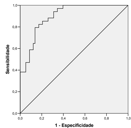
Curva ROC
