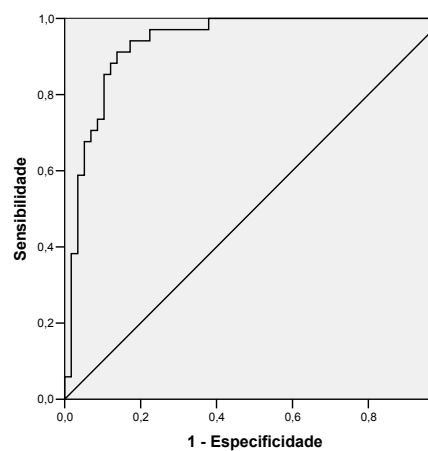
Curva ROC
