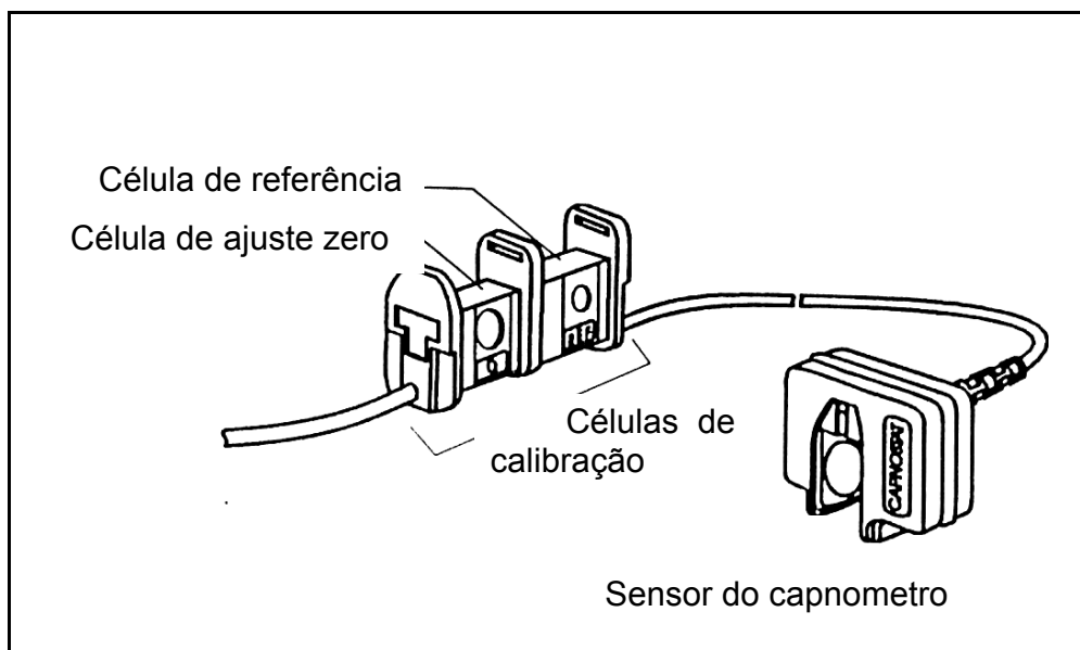
Figura 13 – Capnosat Dixtal/Novametrix®. A sequência de calibração interna está incorporada ao software do aparelho. Duas células de referência são utilizadas para a calibração. A célula zero sem \text{PCO}_2 e a célula de referência com \text{PCO}_2 de 38 mmHg. Embora não necessária, uma segunda calibração externa foi realizada com dois gases de referência certificados pela firma fornecedora de gases (Gás 1: \text{CO}_2 = 20\% e \text{N}_2 = 80\% e Gás 2: \text{CO}_2 = 5\% , \text{O}_2 = 20\% e \text{N}_2 = 75\% ).
