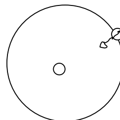
Modelo planetário
