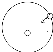
Modelo atômico
