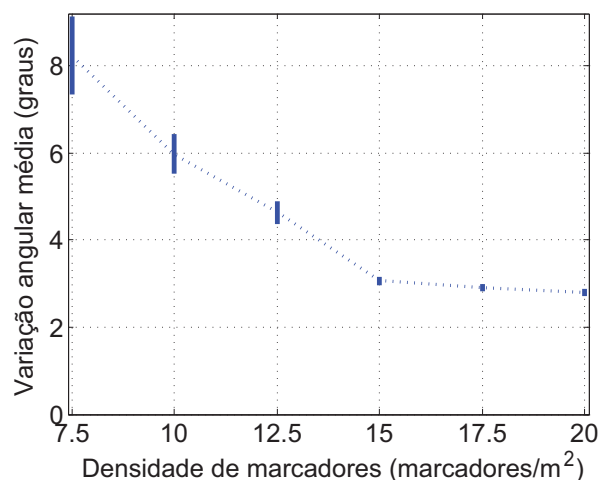
Fig. 5.3: Variação angular média da orientação de um agente a cada iteração na simulação em função da densidade dos marcadores. As barras verticais no gráfico indicam o desvio padrão das médias obtidas nos experimentos para uma mesma densidade de marcadores.
