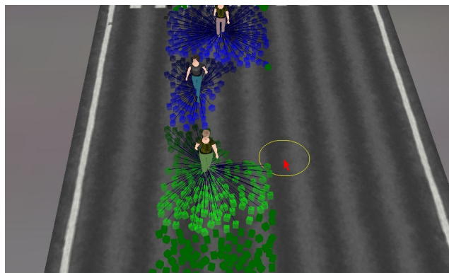
Fig. 6.1: Protótipo desenvolvido no laboratório VHLab/PPGCC/PUCRS que possibilita controlar interativamente a multidão simulada. O usuário pode “pulverizar” marcadores (pontos em verde, no cenário) na superfície. A distribuição e a densidade de marcadores direciona o deslocamento dos agentes.
