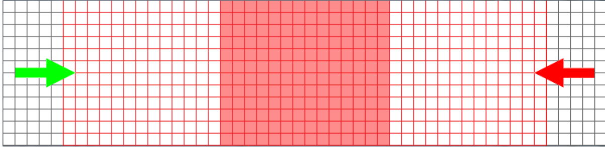
Fig. 5.1: Cenário de simulação utilizado na análise dos principais parâmetros do modelo proposto. As linhas em vermelho na grade indicam a área analisada, sendo que a área central do corredor considerada é a área quadriculada hachurada. As setas indicam o sentido de deslocamento dos grupos de agentes.
