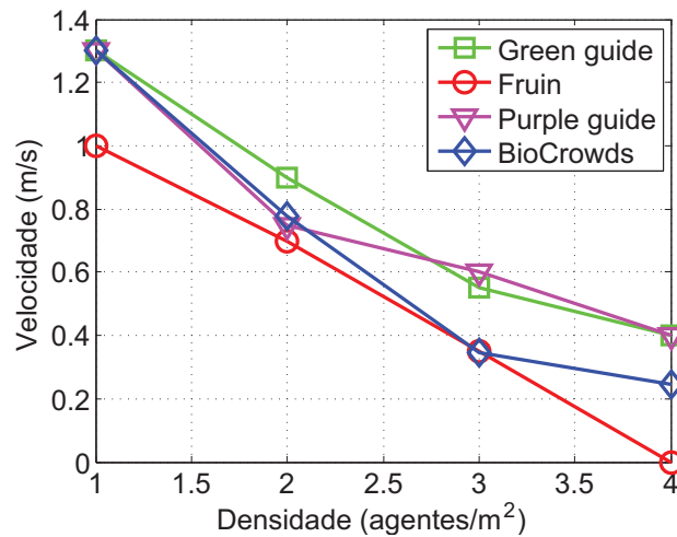
Fig. 5.15: Velocidade média dos agentes como função da densidade populacional local da multidão. Os gráficos referentes ao Green Guide , ao Fruin e ao Purple Guide representam dados medidos de multidões reais, enquanto o gráfico referente ao BioCrowds descreve resultados emergentes apresentados pelo modelo proposto. Nos experimentos realizados, a velocidade máxima dos agentes foi de 1.3 m/s.
