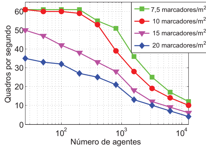
Fig. 5.5: Velocidade de simulação (quadros por segundo) como função da quantidade de agentes, avaliada para quatro densidades de marcadores. Todos os desvios-padrão são menores que um quadro por segundo e, portanto, não são representados graficamente. Os resultados apresentados foram obtidos utilizando somente uma única linha de execução ( monothread implementation ), sem o processo de renderização associado, em um processador Intel® Core™ 2 Duo 2.2GHz e 3GB DDR2 em 667MHz.
