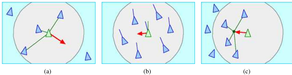
Fig. 2.4: As regras propostas por Reynolds para definir o comportamento coletivo dos boi ds (REYNOLDS, 1987): (a) separação, (b) alinhamento e (c) coesão.
