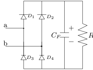
Figura 4.7: Retificador em ponte completa com filtro capacitivo aplicado como carga do sistema UPS mostrado na Figura 4.6.
