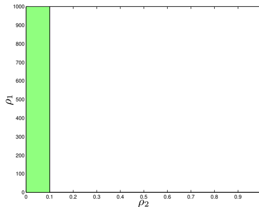
Figura 3.1: Domínio de estabilidade do sistema (2.4) com vértices (3.20) em função dos limitantes das taxas de variação dos parâmetros.
