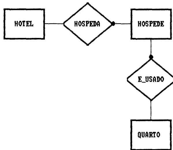
Figura 3.7 - Exemplo da configuração proibida 3.2a.
