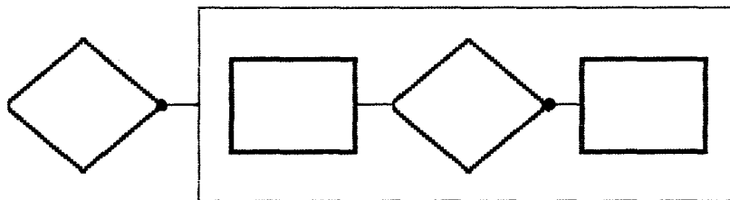
Figura 3.4 - Configuracao Proibida envolvendo Agregacao e Relacionamentos Totais.
