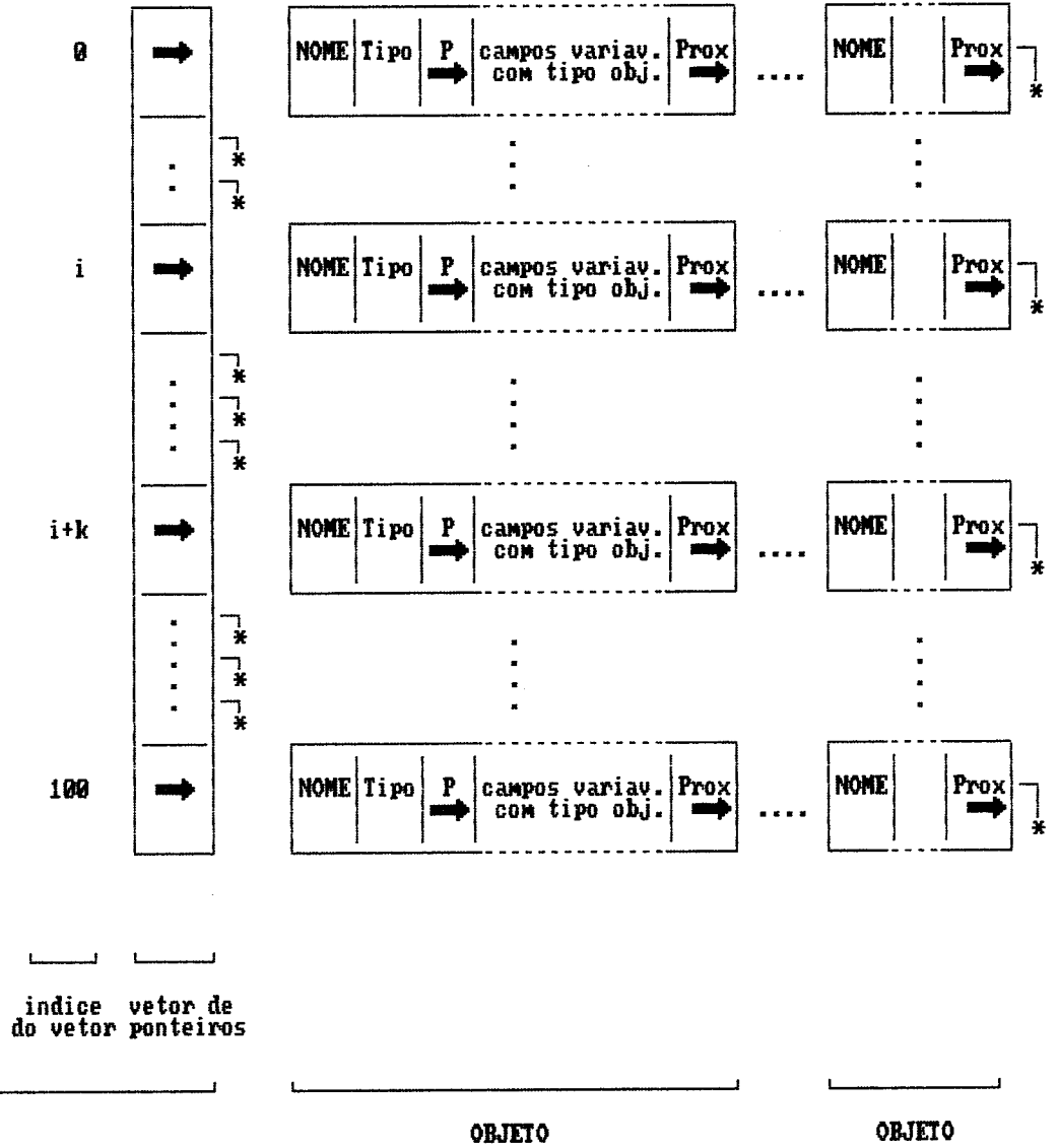
Figura 4.1 - ESTRUTURA INTERMEDIARIA
