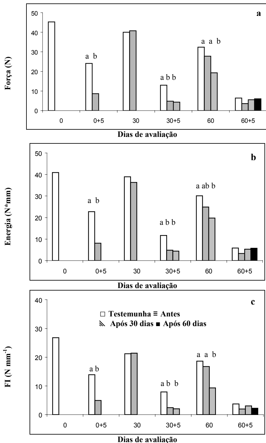
FIGURA 23. Valores médios da Força (a) e Energia (b) necessária para deformação de 3 % do diâmetro do fruto e IF (c) obtidos da compressão de caquis destanzados com CO 2 . Antes, Após 30 dias e Após 60 dias do armazenamento por dois meses. * Letras diferentes sobre as colunas indicam diferenças significativas ( P \leq 0,05 ) segundo Tukey. A ausência de letras indica a não significância. ** + 5 = período de comercialização simulada, onde os frutos permaneceram por 5 dias a 25 \pm 1^\circ\text{C} 80 \pm 5\% UR.
