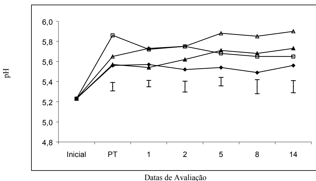
FIGURA 12. pH de caquis 'Rama Forte' durante a destanização com (□) CO 2 , (▲) etanol, (△) etileno e (◆) testemunha e posterior armazenamento a 25°C 90 % de UR durante 14 dias. Inicial = avaliação antes da exposição aos tratamentos, PT = avaliação após o s tratamentos, 1... 14 = avaliação nos respectivos dias de armazenamento a 25°C 90 % UR. Barras no sentido vertical indicam a diferença mínima significativa (DMS) com probabilidade de 5% segundo o teste de Tukey.
