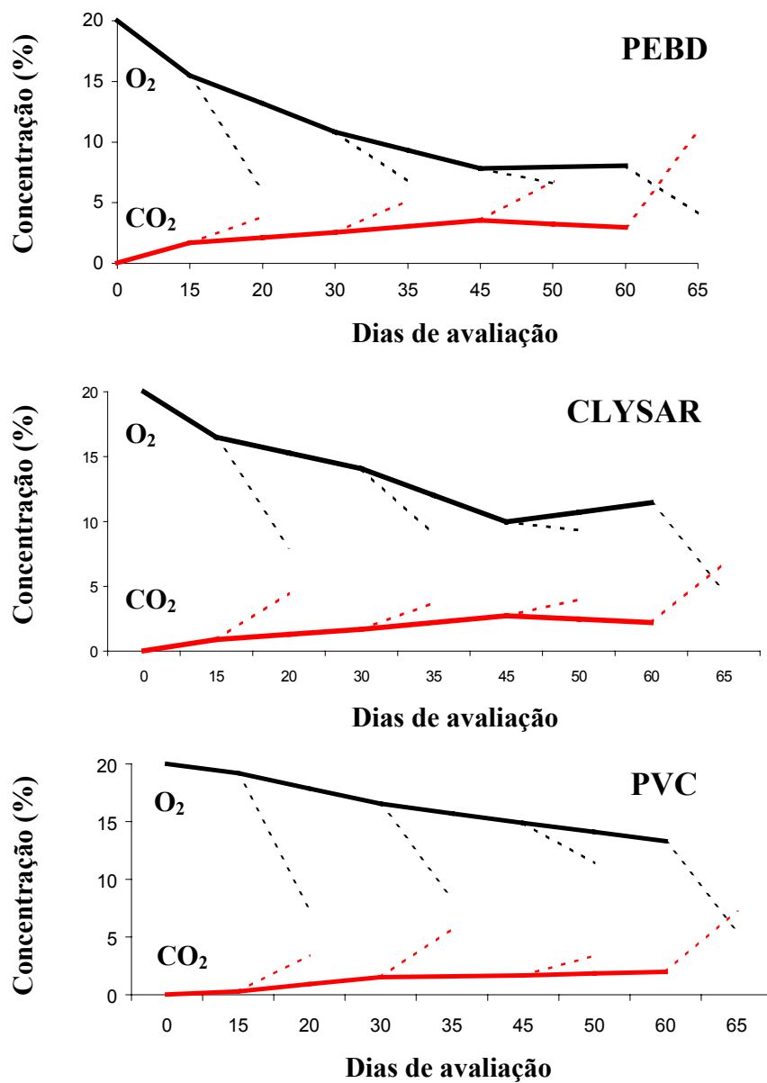
FIGURA 25. Concentrações de O 2 e CO 2 medidos no espaço livre de três diferentes filmes plásticos usados para o acondicionamento de caquis previamente destanizados com CO 2 e armazenados por 60 dias a 1°C 90% UR. Linha contínua (refrigeração) e linha tracejada (comercialização simulada a 25°C).
