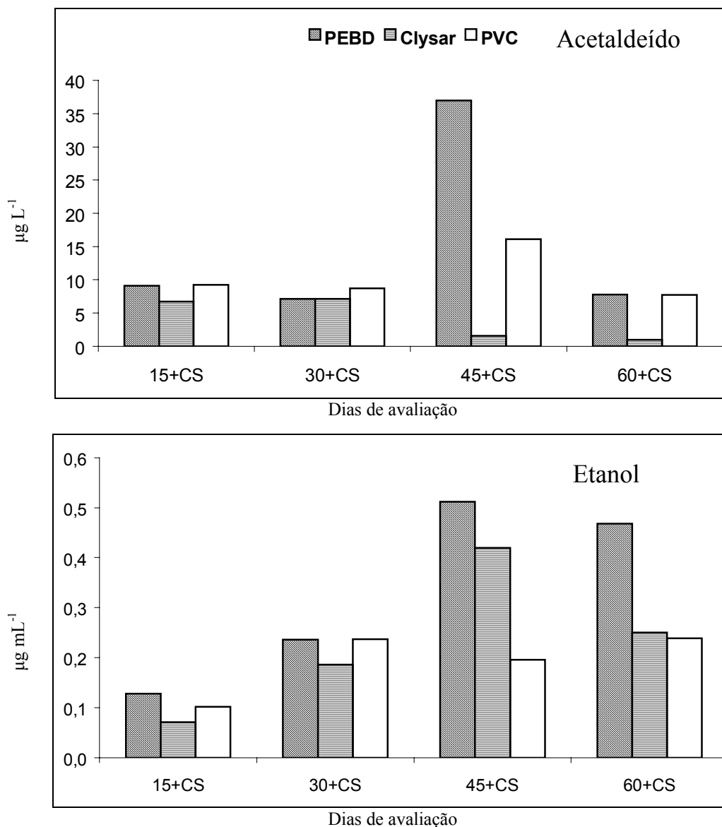
FIGURA 26. Níveis de acetaldeído e etanol medidos em três diferentes embalagens usadas para o acondicionamento de caquis ‘Rama Forte’ previamente destanizados com CO 2 e armazenados por dois meses a 1±1°C 90±5% UR. As análises foram feitas somente após um período de 5 dias de comercialização simulada (CS), onde os frutos permaneceram a 25°C.
