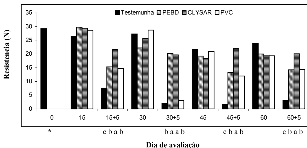
FIGURA 30. Valores médios da resistência da polpa à penetração (N) de caquis ‘Rama Forte’ destanizados com CO 2 e posteriormente acondicionados em três diferentes filmes flexíveis e armazenados por dois meses a 1±1°C 90±5% UR. * Letras diferentes sob as colunas indicam diferenças significativas (P≤0,05) segundo Tukey. A ausência de letras indica a não significância. +5 = período de comercialização simulada, onde os frutos permaneceram por 5 dias a 25±1°C 80±5% UR.
