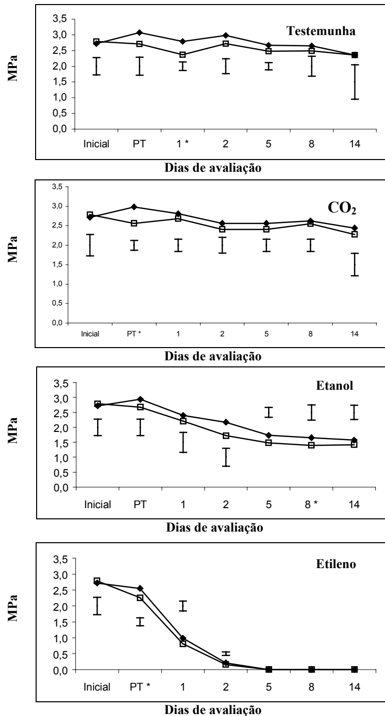
FIGURA 17. Valores médios de módulo de elasticidade obtido das curvas de Tensão-Deformação após a compressão de Espécimes Verticais (♦) e Horizontais (□) extraídos da polpa de caquis após a destanização. Inicial = avaliação antes da destanização, PT = avaliação após os tratamentos, 1... 14 = avaliação nos respectivos dias de armazenamento. Barras no sentido vertical indicam diferença mínima significativa (DMS) ( P \leq 0,05 ) Tukey. * indica diferença significativa.
