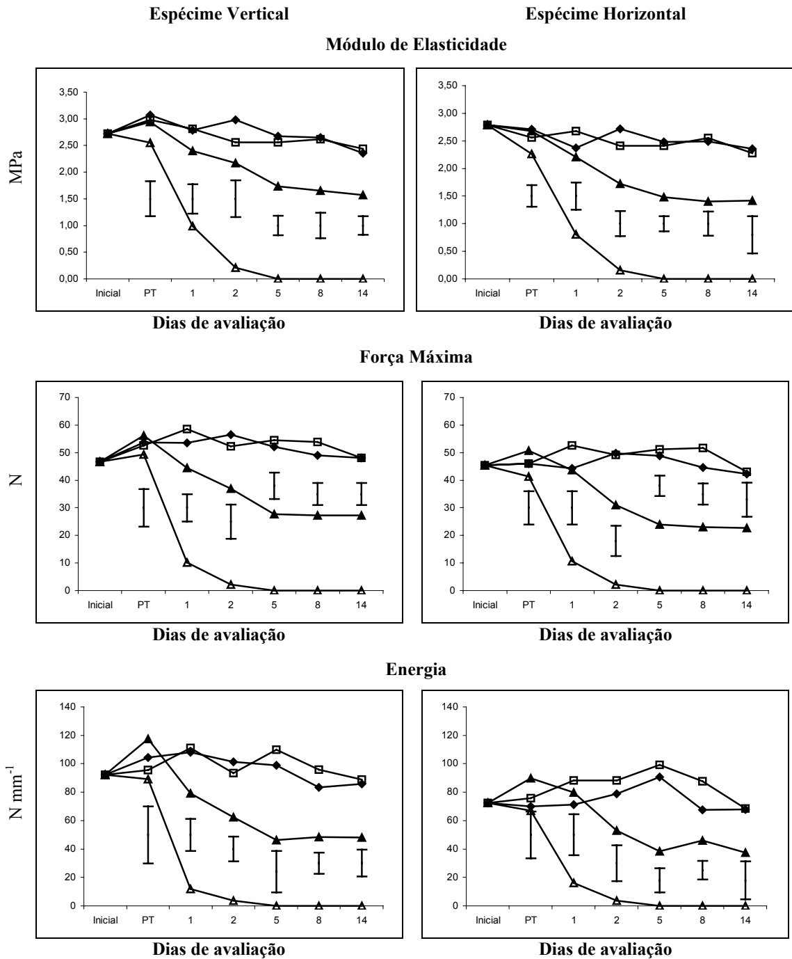
FIGURA 18. Valores médios de Módulo de Elasticidade, Força máxima e Energia requerida para ruptura de espécimes extraídos da polpa de caquis em diferentes processos de destanização com (□) CO 2 , (▲) etanol, (△) etileno e (◆) testemunha. Inicial=avaliação antes da exposição aos tratamentos, PT=avaliação após os tratamentos, 1... 14=avaliação nos respectivos dias de armazenamento. Barras no sentido vertical indicam a diferença mínima significativa (DMS) com probabilidade de 5% segundo o teste de Tukey.
