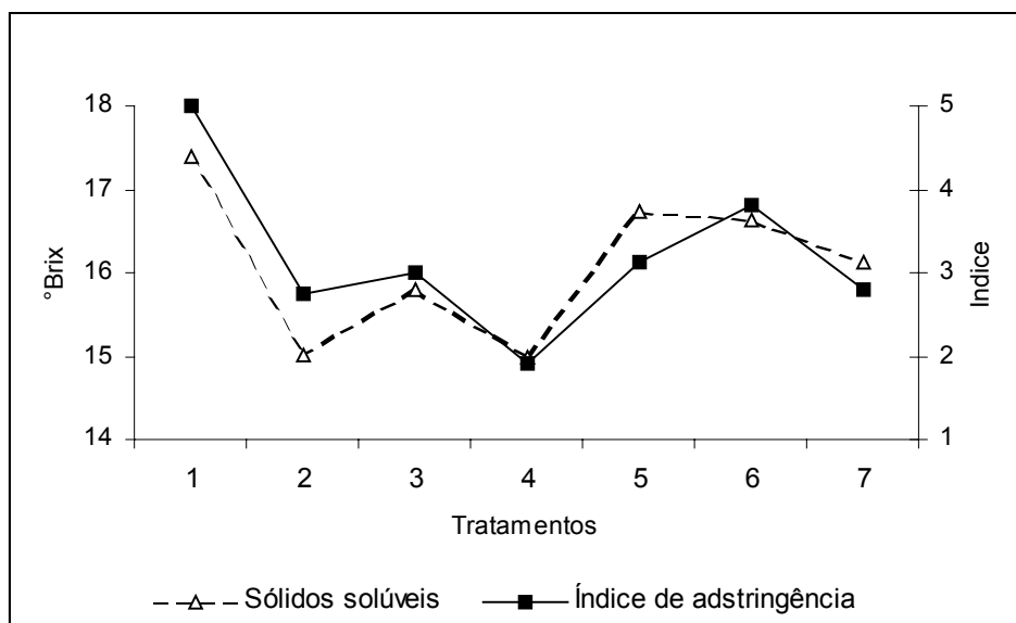
FIGURA 05. Relação entre Sólidos solúveis e Índice de adstringência de caquis 'Rama Forte' após a exposição (Dia 1) a 70 ou 90 % de CO 2 por 12, 18 ou 24 h. Tratamentos: 1 = 0 % / 18 h; 2 = 70 % / 12 h; 3 = 70 % / 18 h; 4 = 70 % / 24 h; 5 = 90 % / 12 h; 6 = 90 % / 18 h e 7 = 90 % / 24 h. Regressão linear significativa ( P \leq 0,05 ), R = 0,87 .
