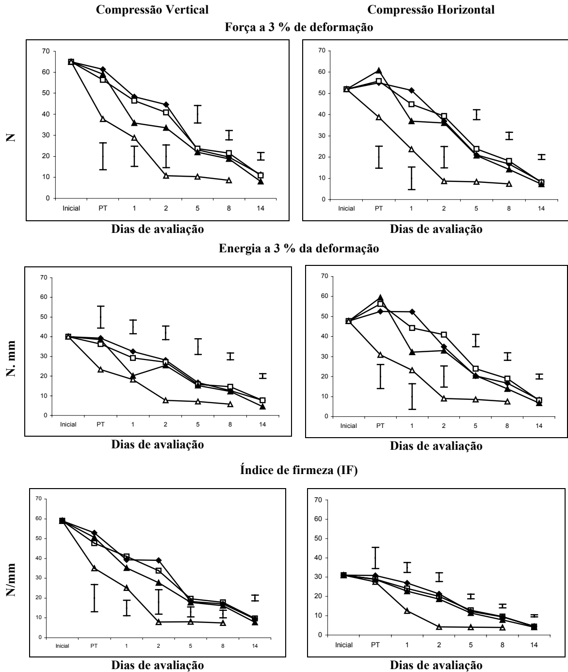
FIGURA 15. Valores médios de Força e Energia necessária para deformação de 3 % do diâmetro do fruto e IF de caquis submetidos à compressão antes e após diferentes processos de destanização com (□) CO 2 , (▲) etanol, (△) etileno e (◆) testemunha. Inicial = avaliação antes da exposição aos tratamentos, PT = avaliação após os tratamentos, 1... 14 = avaliação nos respectivos dias. Barras verticais indicam a diferença mínima significativa (DMS) segundo o teste de Tukey a P \leq 0,05 .
