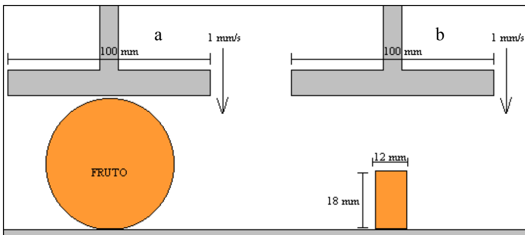
FIGURA 07. Compressão entre pratos planos, rígidos e paralelos do Fruto Inteiro (a) e espécimes cilíndricos (b).
