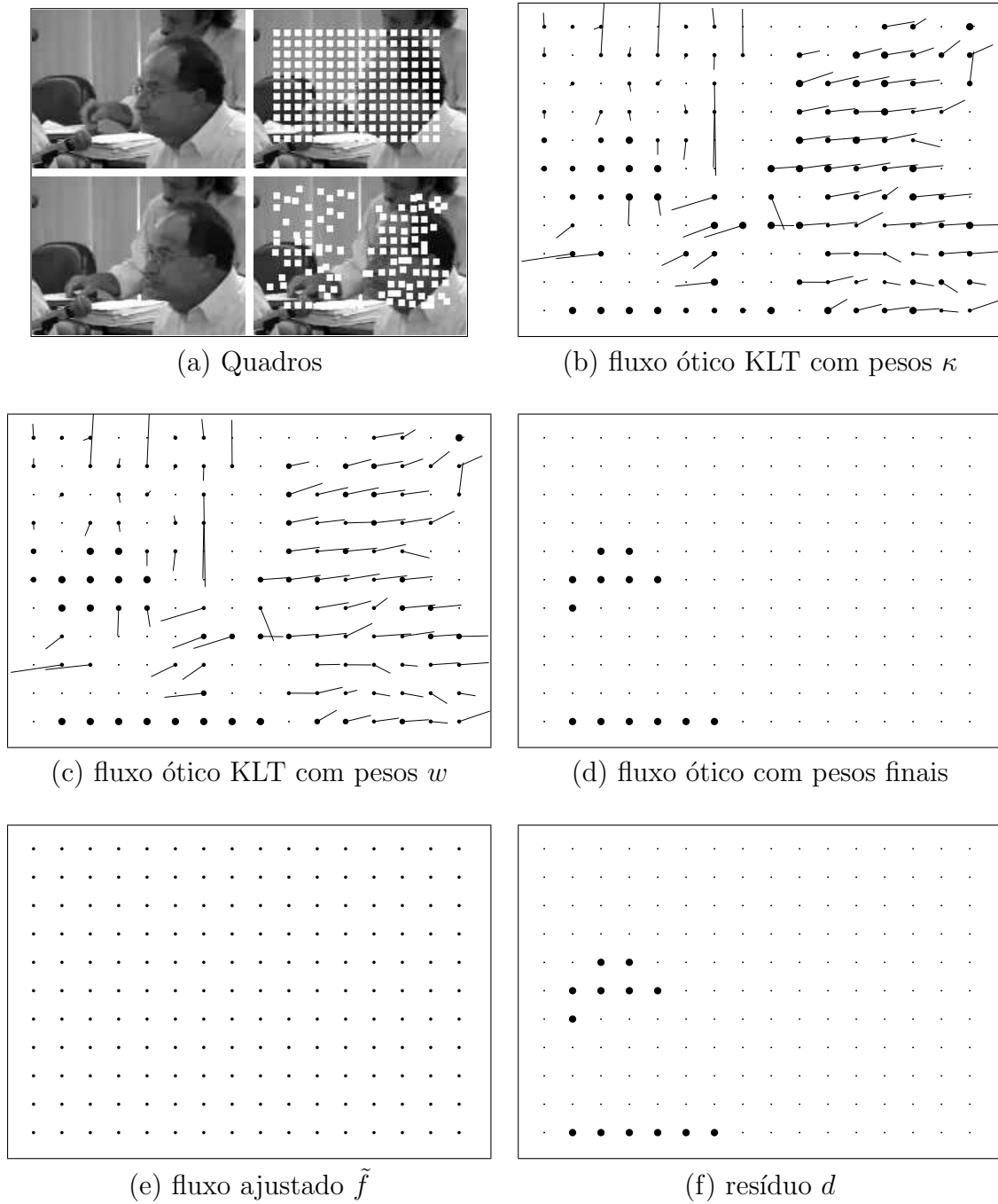
Figura 7.3: Resultado do algoritmo WOFF completo aplicado a dois quadros consecutivos do vídeo consu2 .
