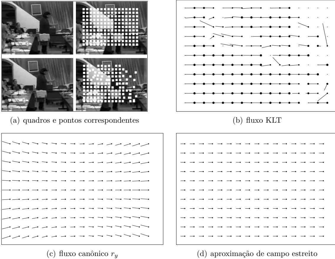
Figura 4.5: Fluxos óticos devidos a movimento de pan.
