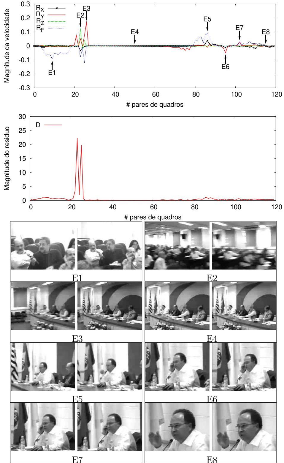
Figura 6.3: Outro gráfico com variações das velocidades de R_x , R_y , R_z , R_f , resíduo D e oito eventos selecionados de um segmento com 240 quadros do vídeo consu3 .
