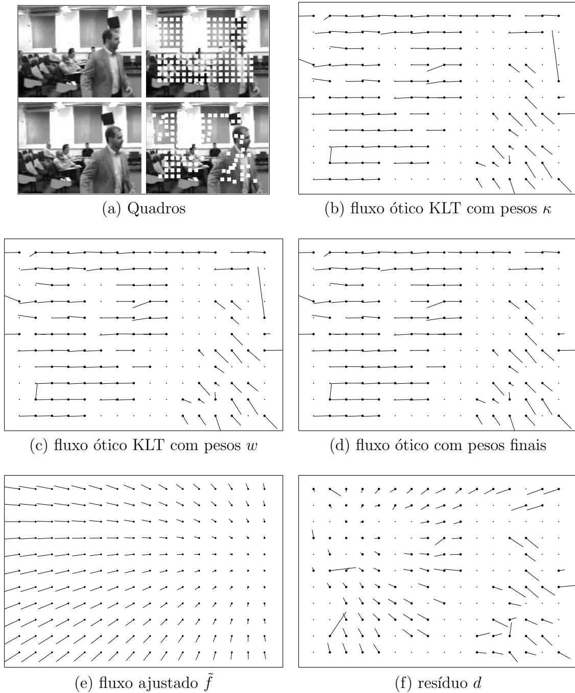
Figura 7.6: Resultados do algoritmo WOFF ignorando os escores de confiabilidade do algoritmo KLT, para os mesmos quadros da figura 7.5.
