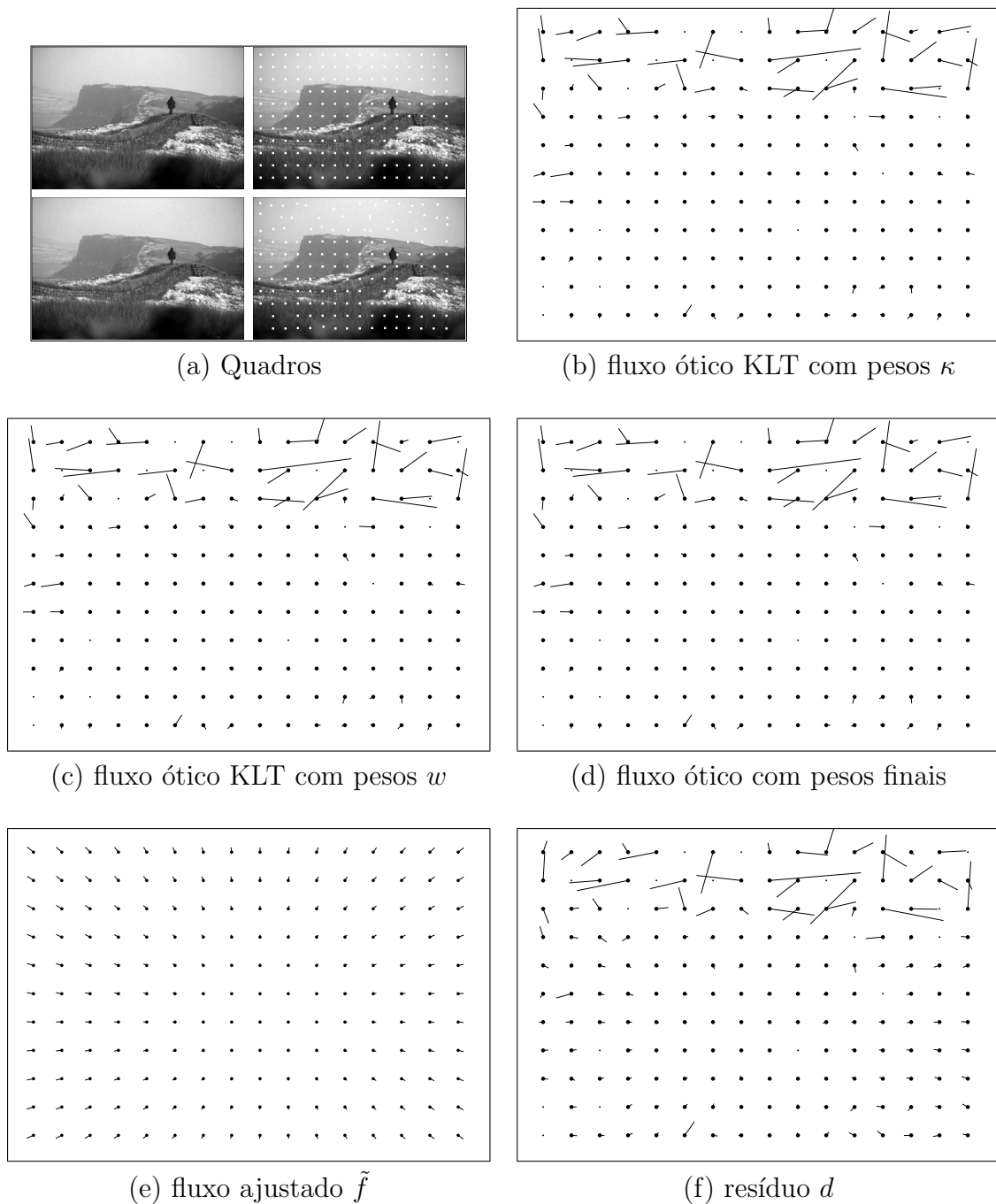
Figura 7.2: Resultados de uma versão do WOFF sem pesos iniciais, sem ajuste inicial dos pesos e sem o ajuste iterativo de pesos, para os mesmos quadros da figura 7.1.
