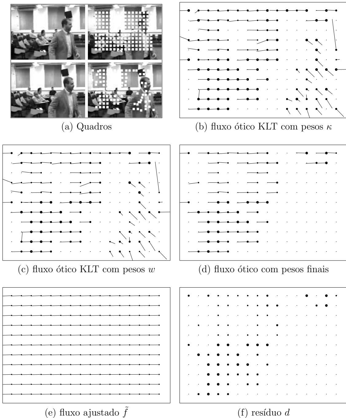
Figura 7.5: Resultado do algoritmo WOFF completo aplicado a dois quadros consecutivos do vídeo consu3 , com escores de confiabilidade \kappa_i fornecidos pelo algoritmo KLT.
