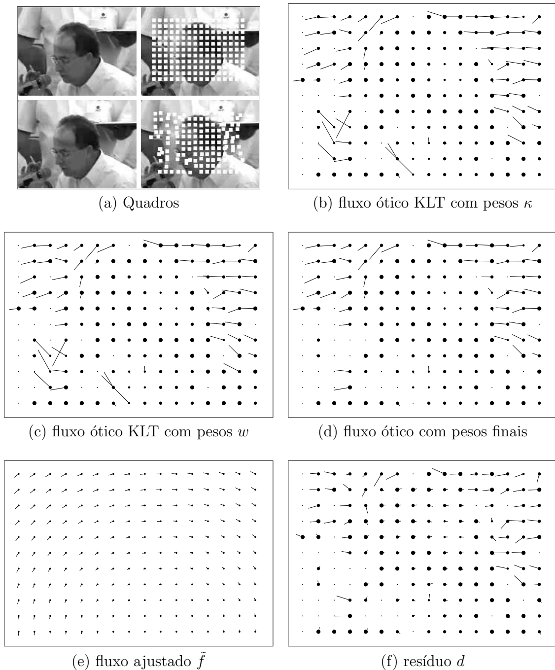
Figura 7.8: Resultados de uma versão do WOFF sem ajuste inicial dos pesos, para os mesmos quadros da figura 7.7.
