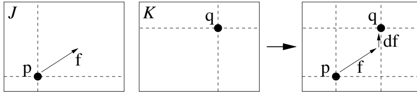
Figura 3.3: Problema de ajuste infinitesimal de deslocamento ótico: dados p e f , tal que J(p) \approx K(p + f) , encontrar um deslocamento pequeno df tal que J(p) \approx K(p + f + df) .
