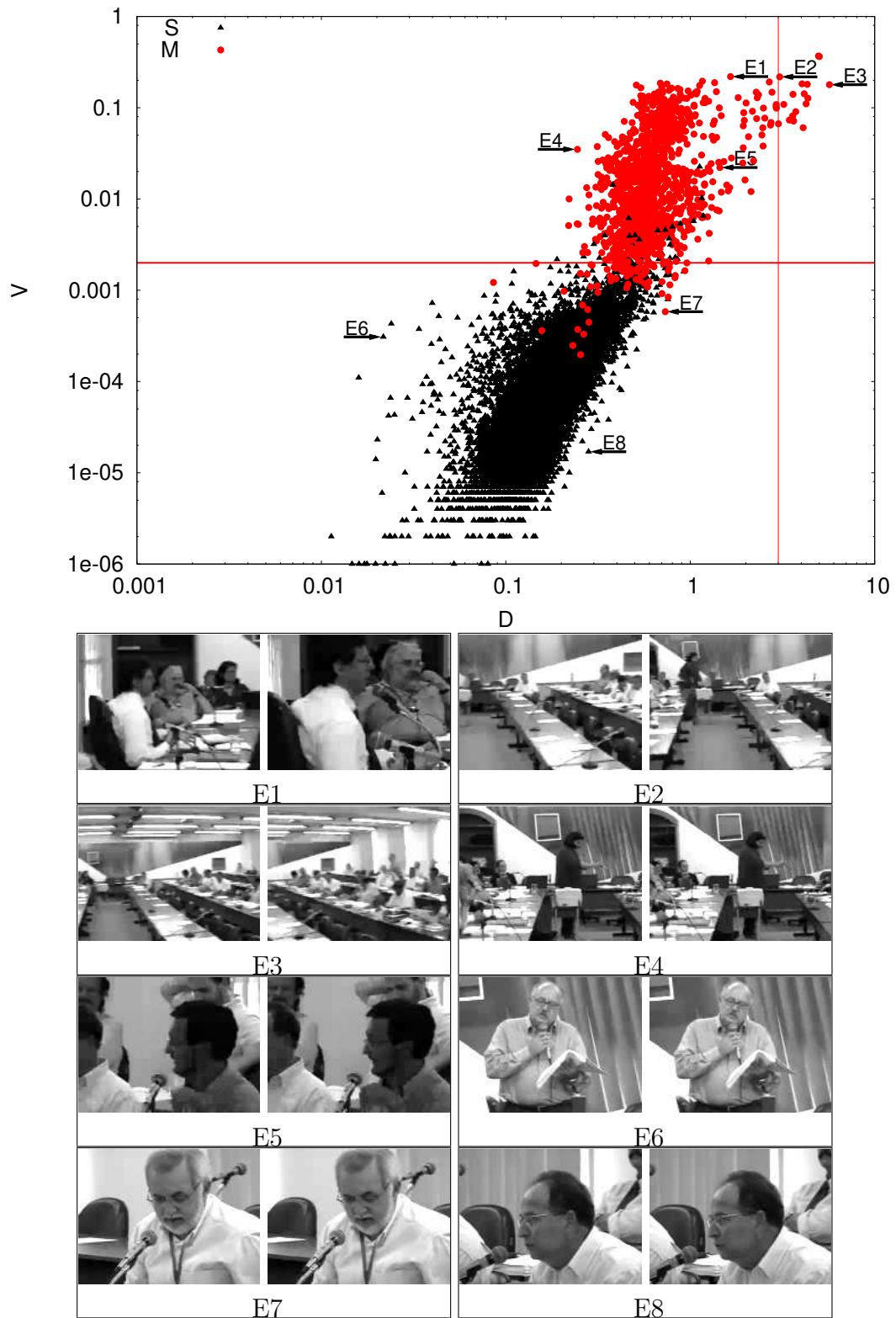
Figura 6.8: Gráfico da velocidade de câmera estimada V pelo erro residual D para todos os pares de quadro do consu1 . Os pares de quadros do tipo S (câmera estacionária) e M (câmera em movimento) são representados por triângulos e círculos, respectivamente. Oito eventos, indicados por setas, mostram o que representam.
