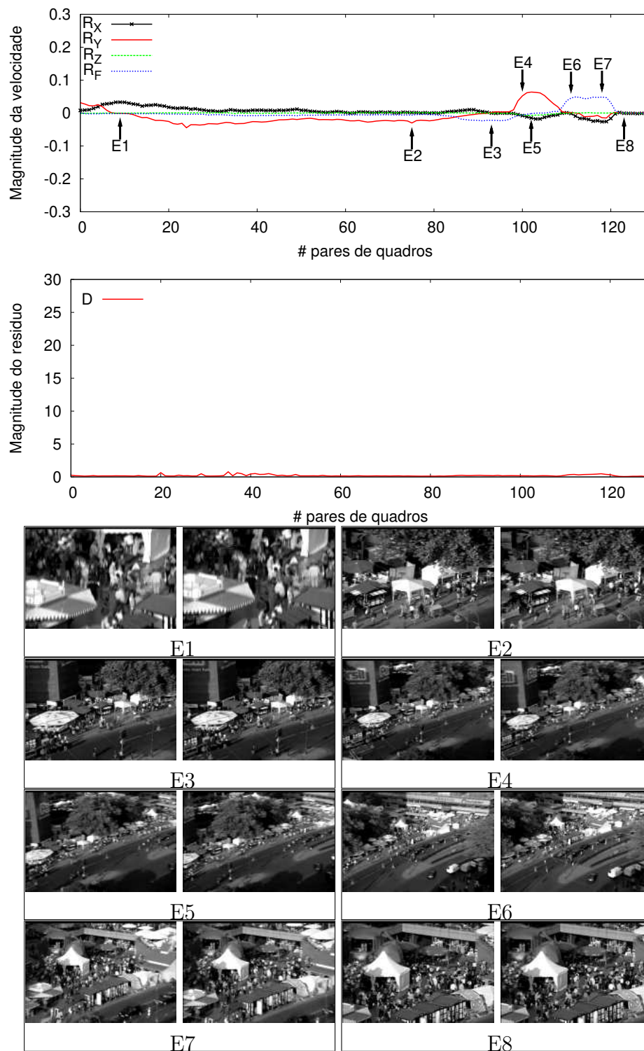
Figura 6.4: Outro gráfico com variações das velocidades de R_x , R_y , R_z , R_f e resíduo D do vídeo feira na íntegra, e oito eventos selecionados.
