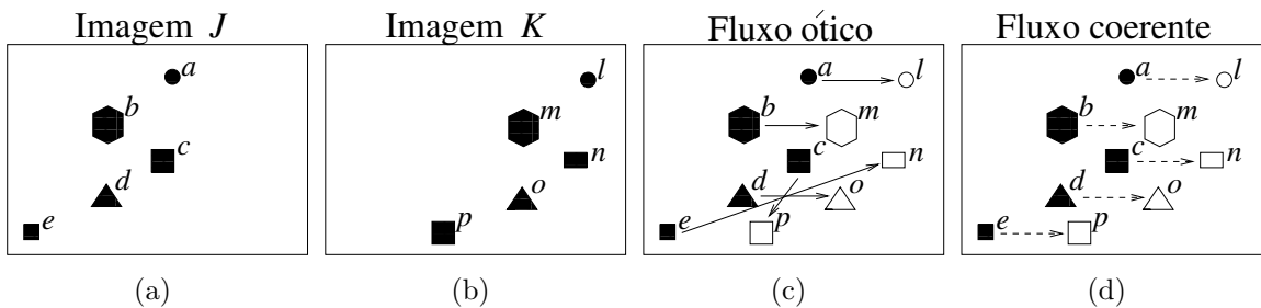
Figura 2.6: Incoerência espacial do fluxo ótico.
