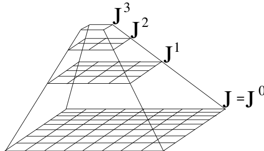
Figura 3.6: Uma pirâmide de imagens para o algoritmo KLT.
