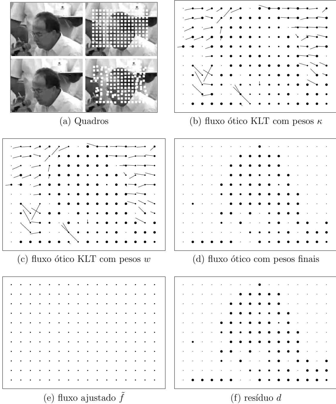
Figura 7.7: Resultado do algoritmo WOFF completo aplicado em dois quadros consecutivos do vídeo consul .
