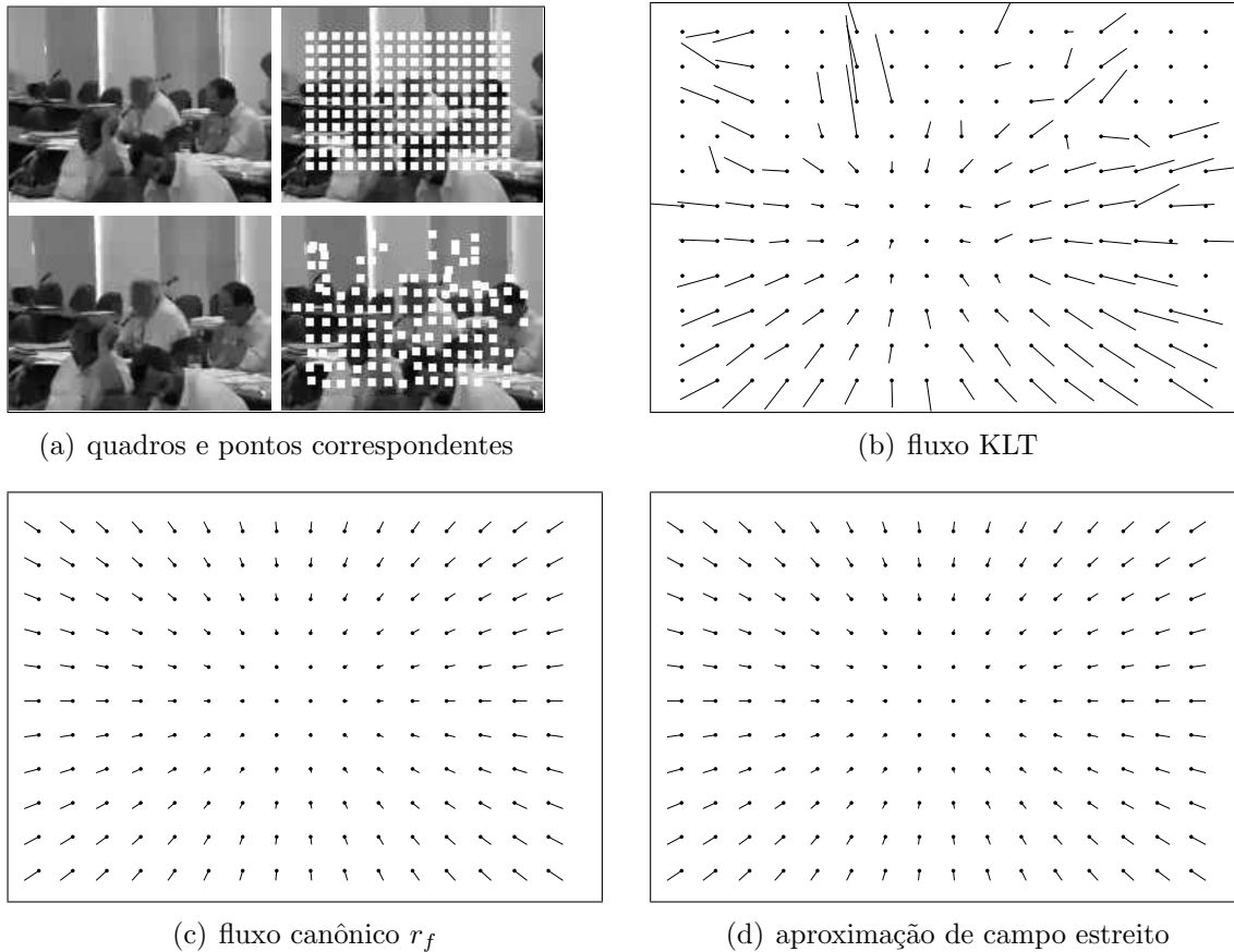
Figura 4.7: Fluxos óticos devidos a movimento de zoom.
