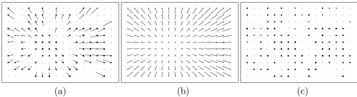
Figura 5.3: Exemplo da análise de mínimos quadrados de um fluxo observado durante uma combinação de zoom-out e pan para a direita; (a) um fluxo alinhado f , com os pesos w_i indicados pelo tamanho dos pontos; (b) fluxo \tilde{f} ajustado a f pelo método dos mínimos quadrados ponderados; (c) resíduo d = f - \tilde{f} .
