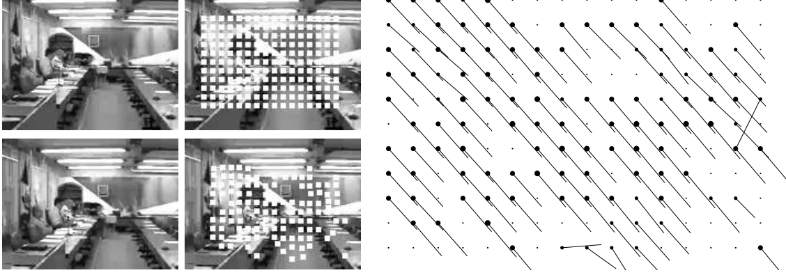
Figura 5.1: Fluxo ótico em um vídeo do Conselho Universitário da Unicamp. Na primeira coluna são mostrados dois quadros consecutivos do vídeo. Na coluna do meio são indicados por quadrados brancos os pontos de amostragem p_1, p_2, \dots, p_n (imagem no alto) e os pontos correspondentes p_i + f(p_i) rastreados pelo algoritmo KLT (imagem de baixo). A figura à direita mostra os vetores f_1, f_2, \dots, f_n (traços) e os pesos w_1, w_2, \dots, w_n (círculos negros).
