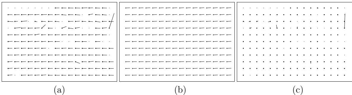
Figura 5.2: Exemplo da análise de mínimos quadrados para o fluxo observado durante um pan da câmera; (a) um fluxo amostrado f , com os pesos w_i indicados pelo tamanho dos pontos; (b) fluxo \tilde{f} ajustado a f pelo método dos mínimos quadrados ponderados; (c) resíduo d = f - \tilde{f} .
