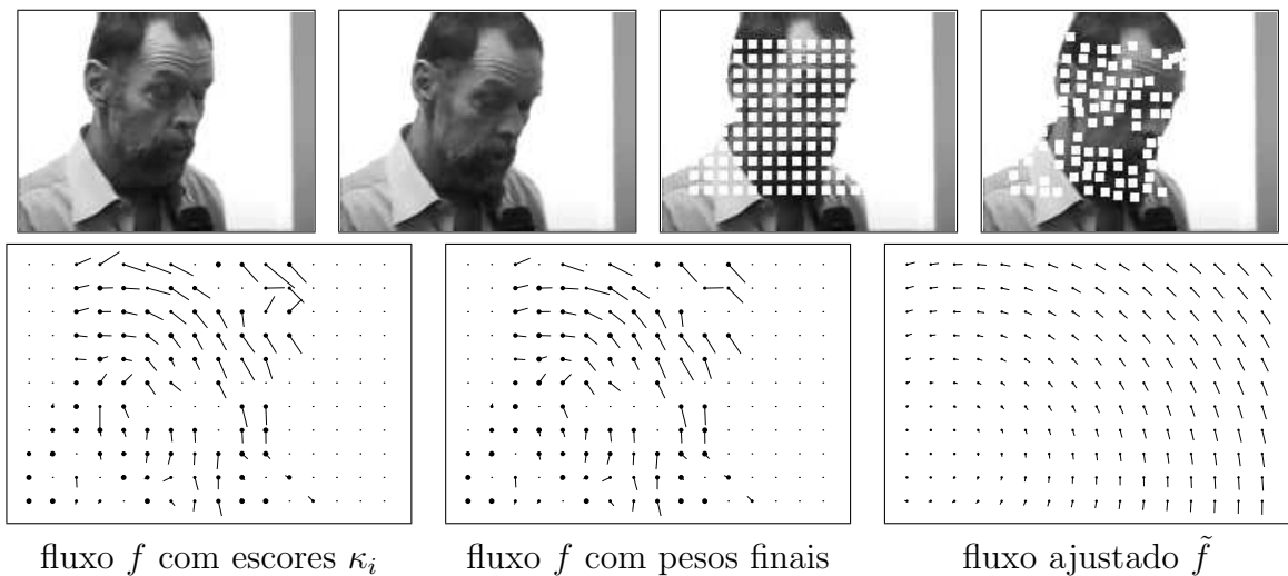
Figura 6.5: Movimento em cena estática pobre em textura causa análise incorreta do fluxo.
