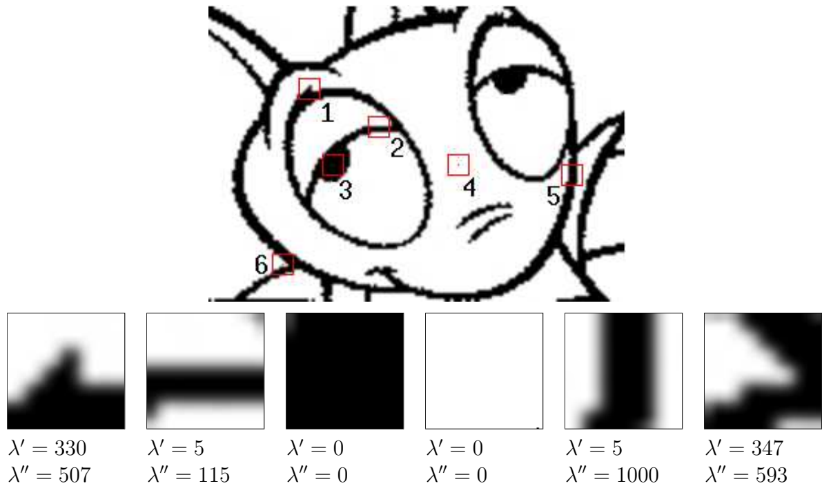
Figura 3.5: Confiabilidade de rastreamento: seis pontos selecionados de uma imagem, (no alto), suas vizinhanças (meio), e os autovalores \lambda' e \lambda'' da matriz G (embaixo).
