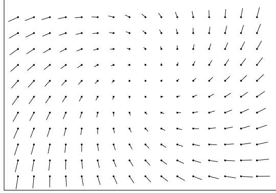
Figura 4.3: Fluxo óptico previsto para movimento de câmera com T_x^* = T_z^* = 0 , T_y^* = Z = 1 , R_y^* = -1 , R_x^* = R_z^* = -2 , R_f^* = 2 e F = 7 .
