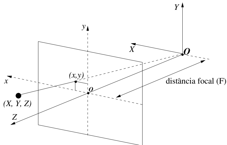
Figura 4.1: O sistema canônico para projeção perspectiva plana.
