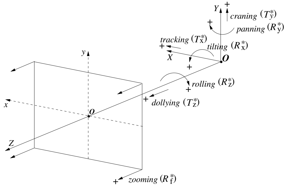
Figura 4.2: Velocidades que definem o movimento instantâneo da câmera.
