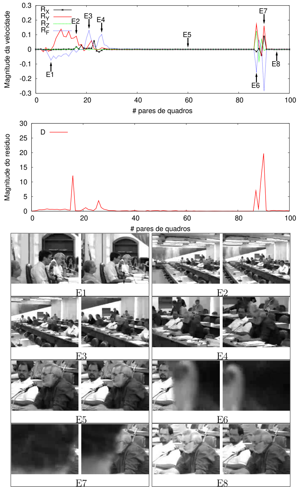
Figura 6.2: No primeiro gráfico são mostradas as variações das velocidades de R_x , R_y , R_z e R_f para um segmento com 200 quadros do vídeo consu2 (100 pares). As amplitudes em cada uma das curvas indica o movimento referido tal como pode ser visto nos eventos E1—E8. O segundo gráfico mostra o residuo D = \|d\| = \|f - \tilde{f}\| em cada análise.
