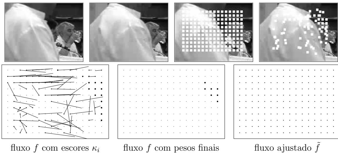
Figura 6.6: Movimento de cena produzindo fluxo caótico, cujos vetores são eliminados no ajuste iterativo.
