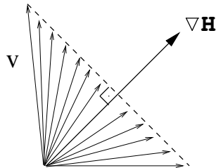
Figura 3.4: Explicação geométrica para a equação de restrição do fluxo ótico. Se algum dos vetores v indicados satisfaz a equação (3.4), então todos eles satisfazem.
