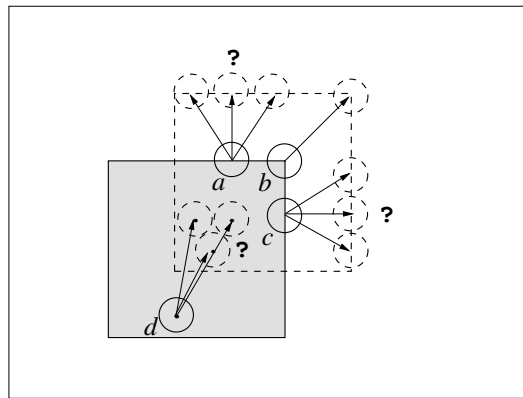
Figura 2.4: Ambigüidade do fluxo ótico.
