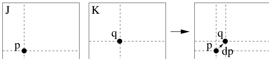
Figura 3.2: Problema de cálculo do deslocamento infinitesimal: dado p , calcular um deslocamento pequeno dp tal que J(p) \approx K(p + dp) .
