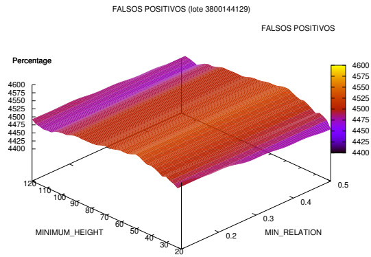
Figura 4.25: Padrão 20, observado em gráficos de falsos positivos da análise conjunta dos parâmetros MINIMUM_HEIGHT e MIN_RELATION.
