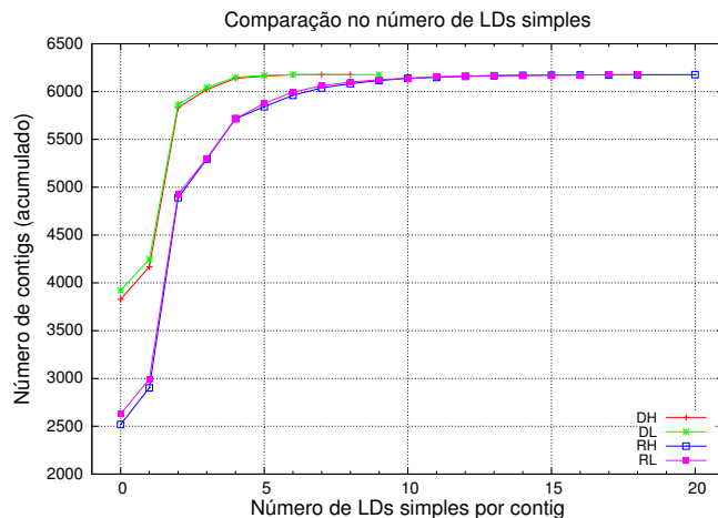
Figura 5.6: Gráfico comparando o número de LDs simples nos diversos casos estudados. No eixo X temos o número de vértices que possuem clique máxima de tamanho dois (LDs simples) por contig e no eixo Y temos o número de contigs . A curva DH representa o caso onde ocorre LD quando D' = 1 e bases de baixa qualidade são excluídas. A curva DL, quando D' = 1 e bases de baixa qualidade são consideradas. A curva RH representa o caso onde ocorre LD quando r^2 \geq 1/3 e bases de baixa qualidade são excluídas. A curva RL, quando r^2 \geq 1/3 e bases de baixa qualidade são consideradas.
