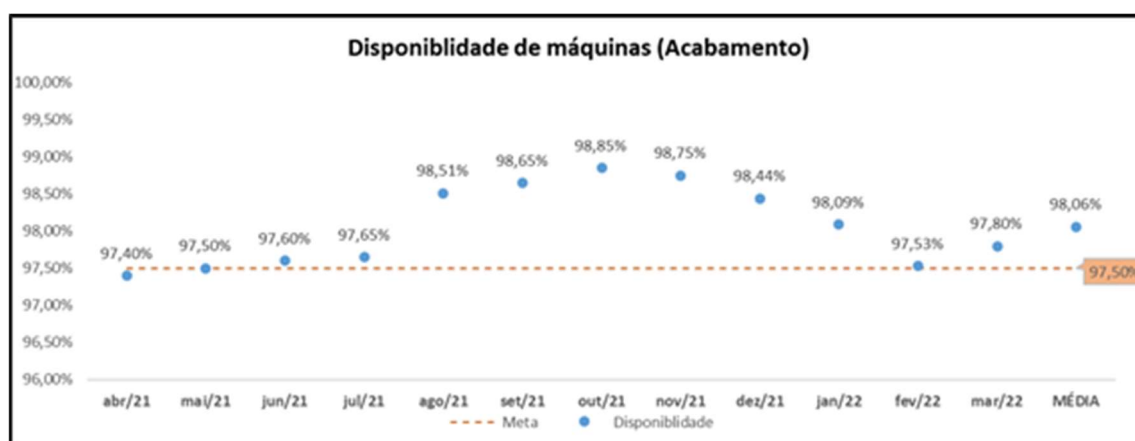
Figura 4 - Indicador de disponibilidade de máquinas (acabamento).
