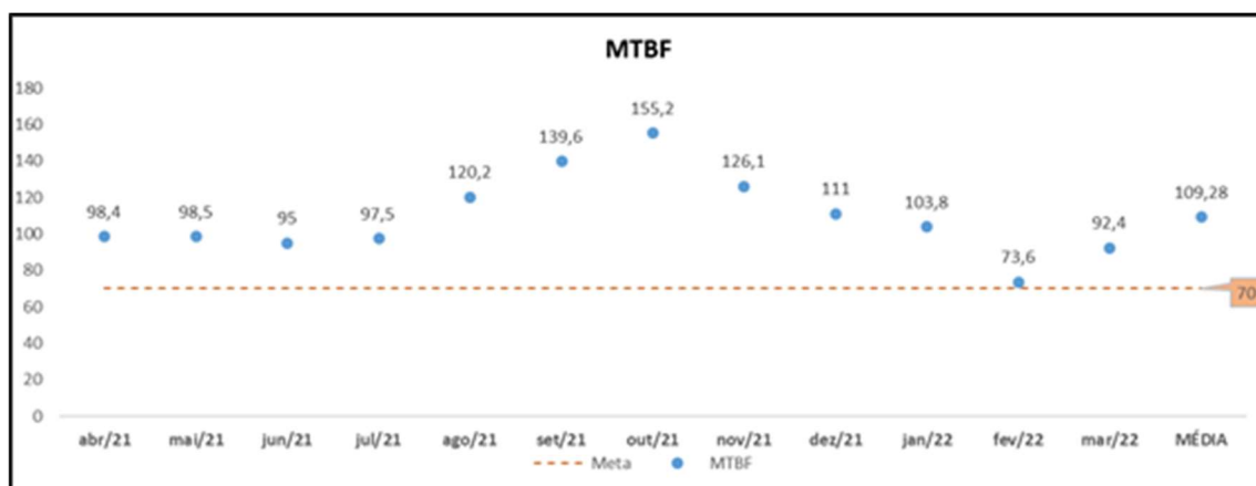
Figura 6 - Indicador MTBF em atuação preventiva nas grandes perdas.
